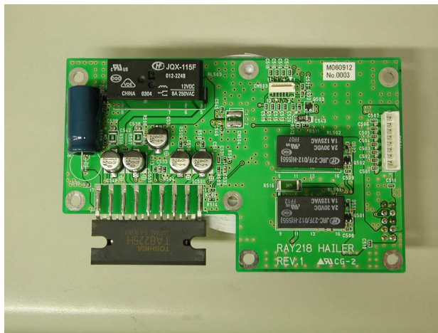
Hailer PCB-1
