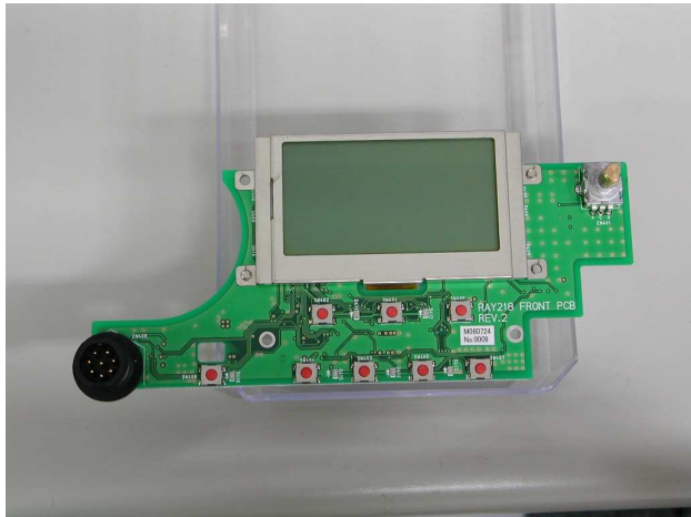
CONT PCB-1
