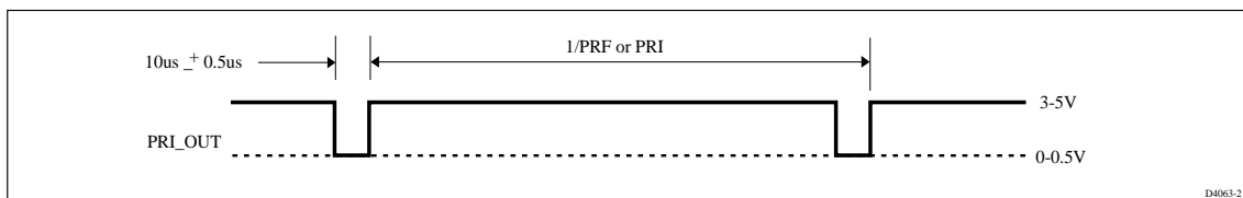
Figure 10: PRI_OUT/PRI_DPOS
