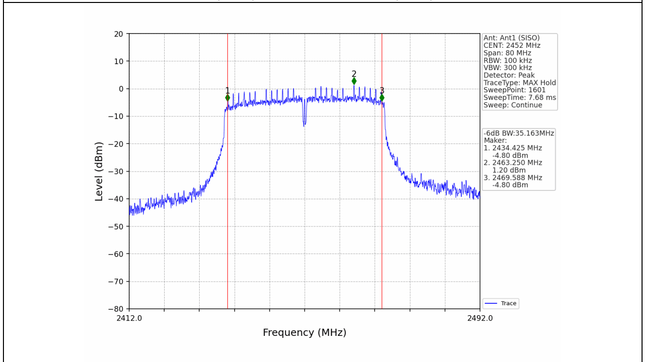
802.11n(HT40)_HCH_2452MHz_Ant1 (SISO)_NTNV
