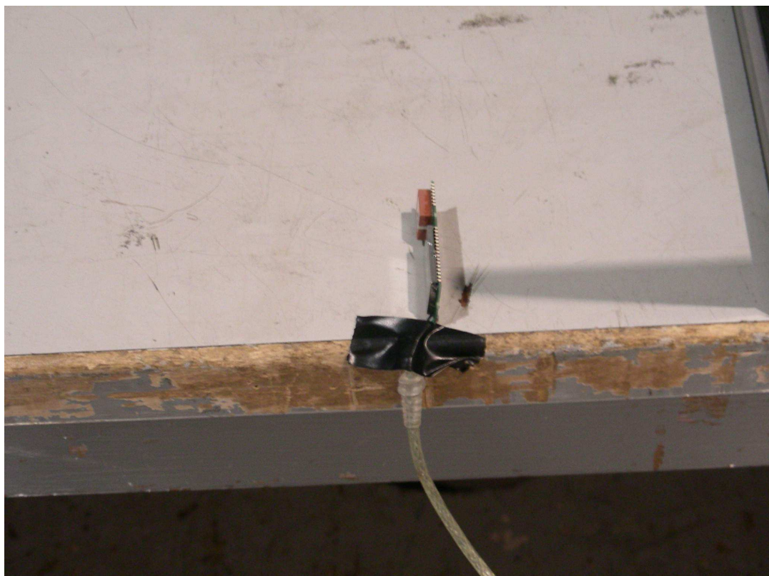
z-axis
