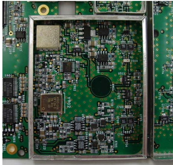
VCO area
