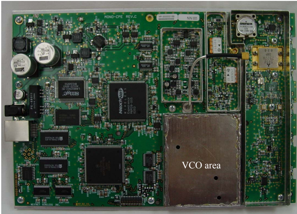
VCO area
