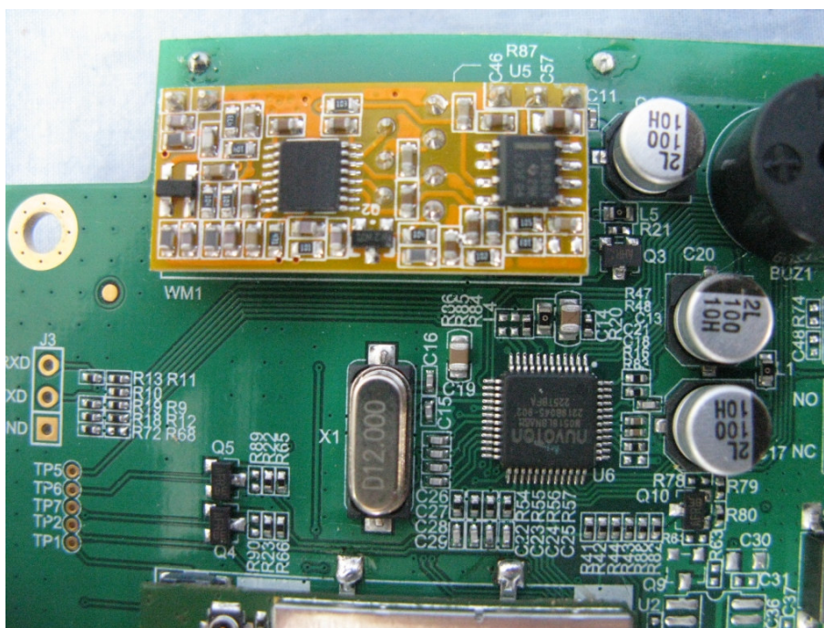
433MHz module
