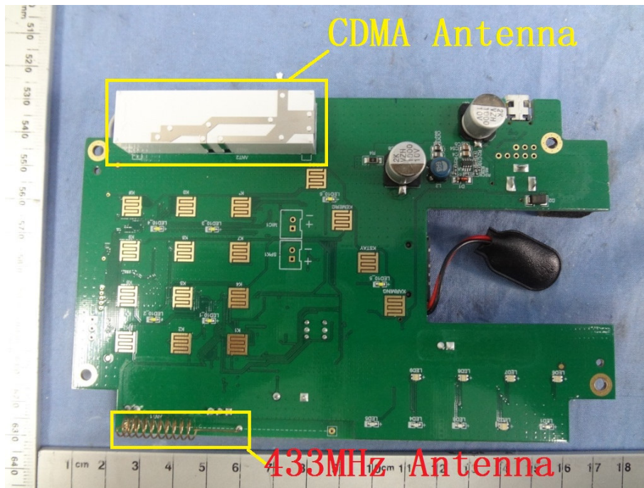
CDMA module
