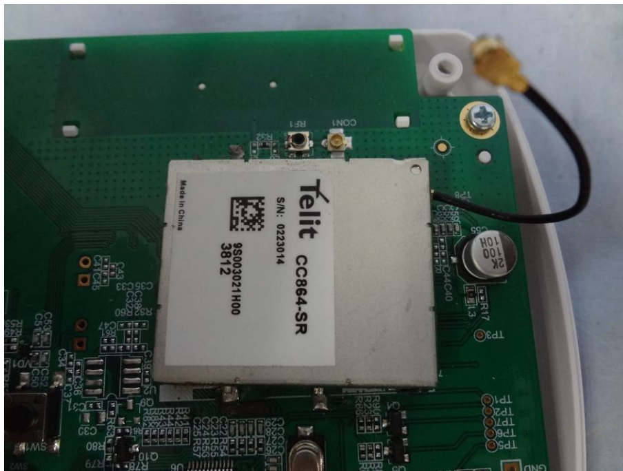
CDMA module
