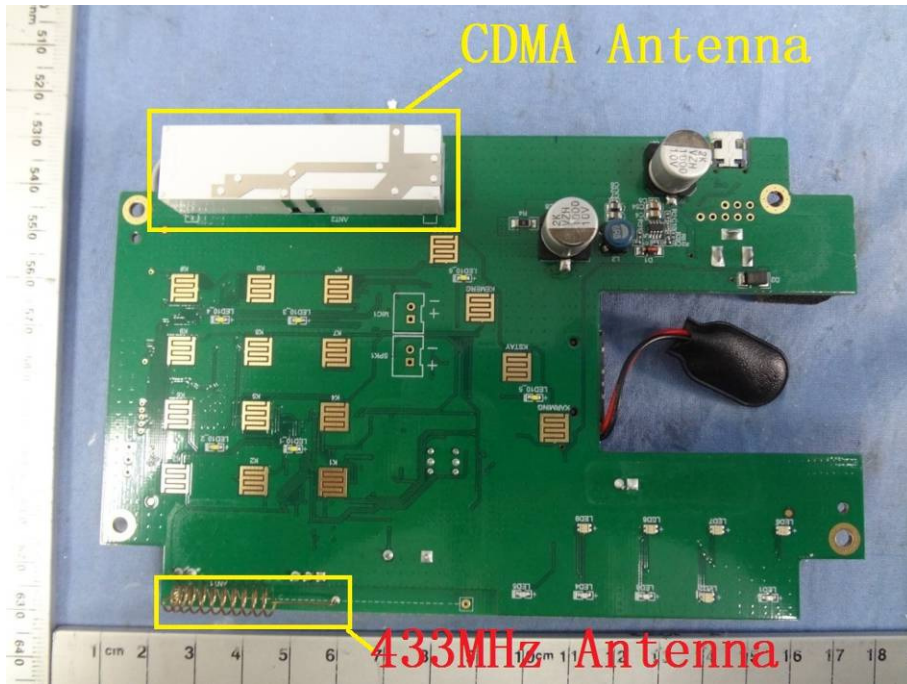
CDMA module
