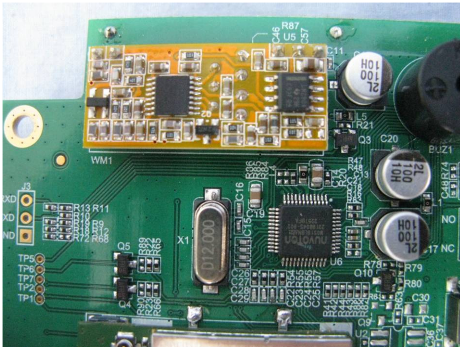
433MHz module
