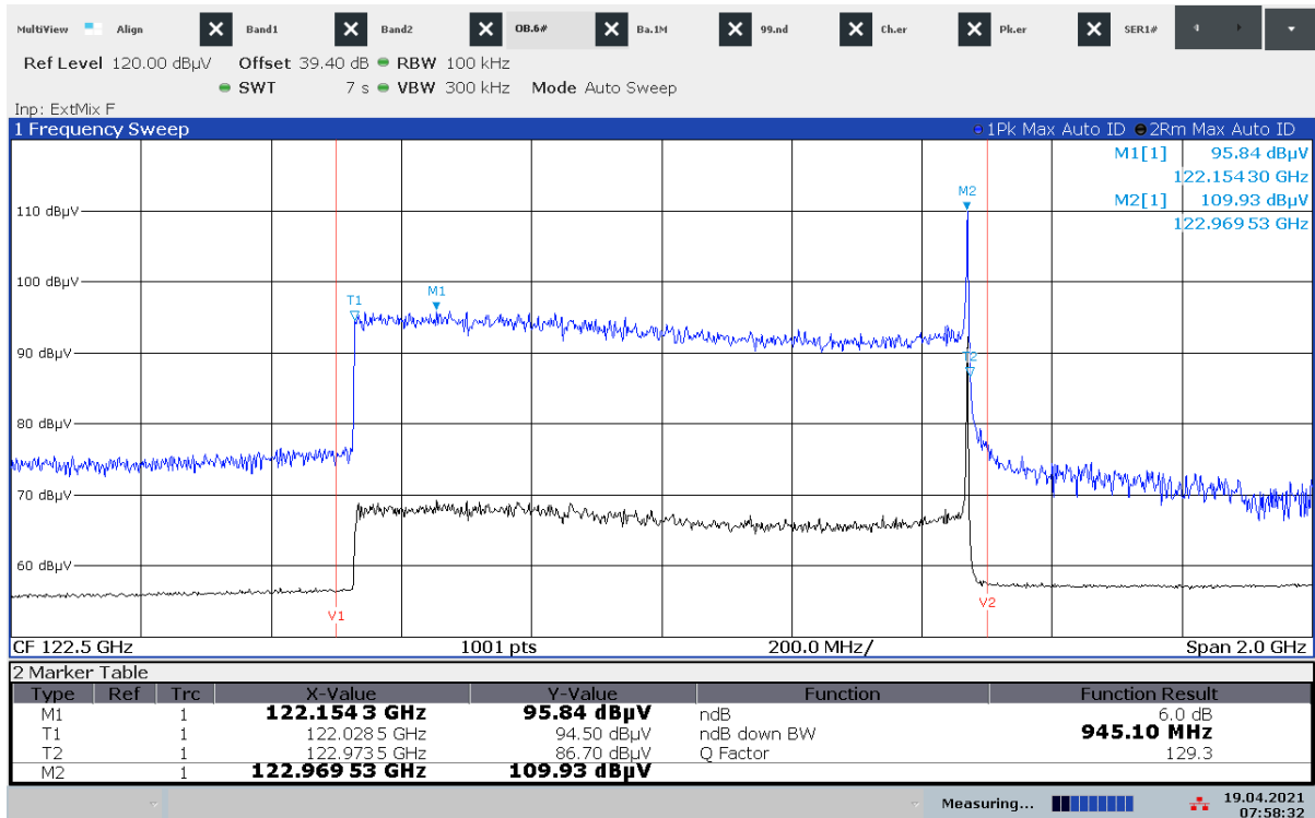
Plot 35: T_{max} / V_{nom}
