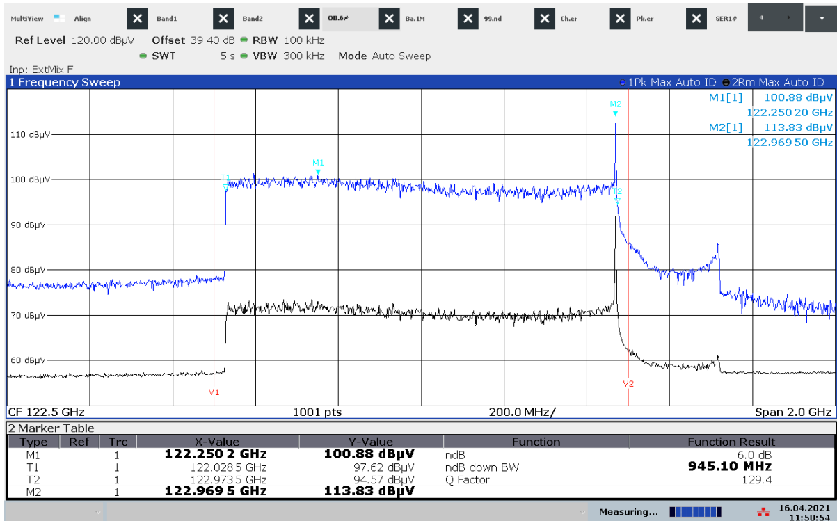
Plot 43: T_{nom} / V_{max}
