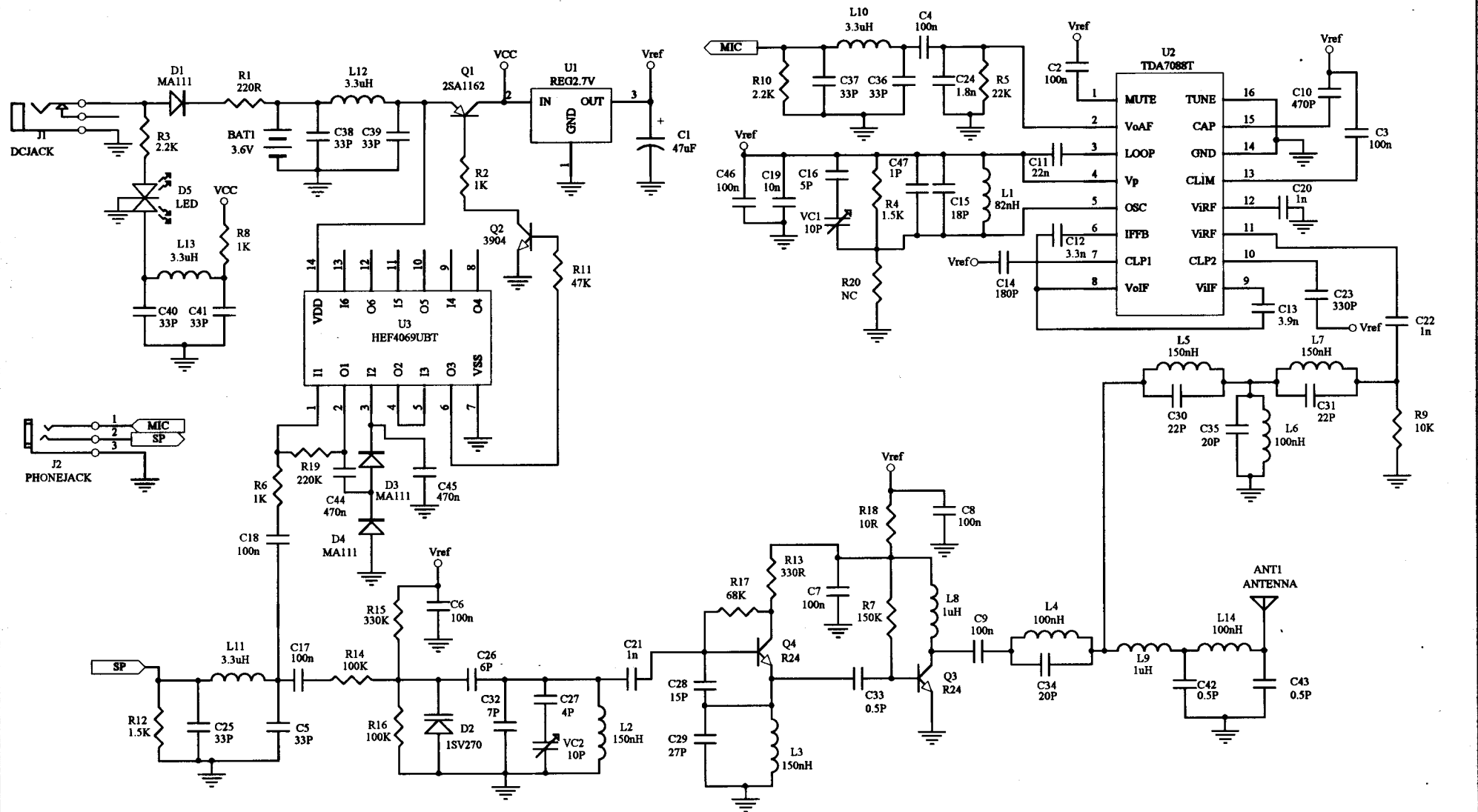
FM HANDFREE 大哥大端(TX 88MHz) (更新日期2001/1/2)
