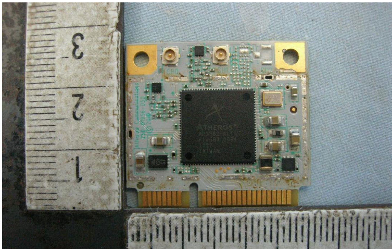
WLAN-121N module_front
