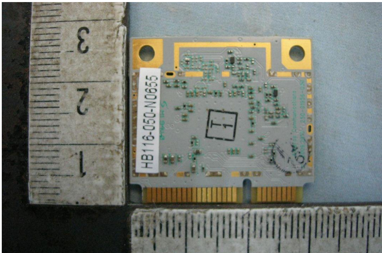
WLAN-121N module_back
