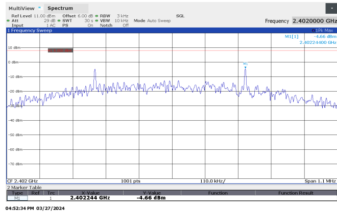
BLE 500 Kbps
