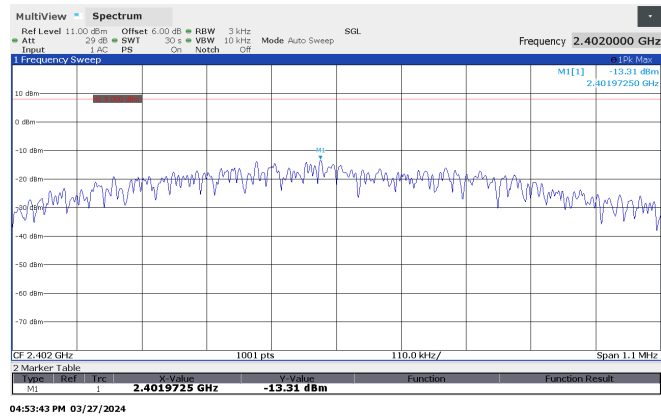
BLE 1Mbps
