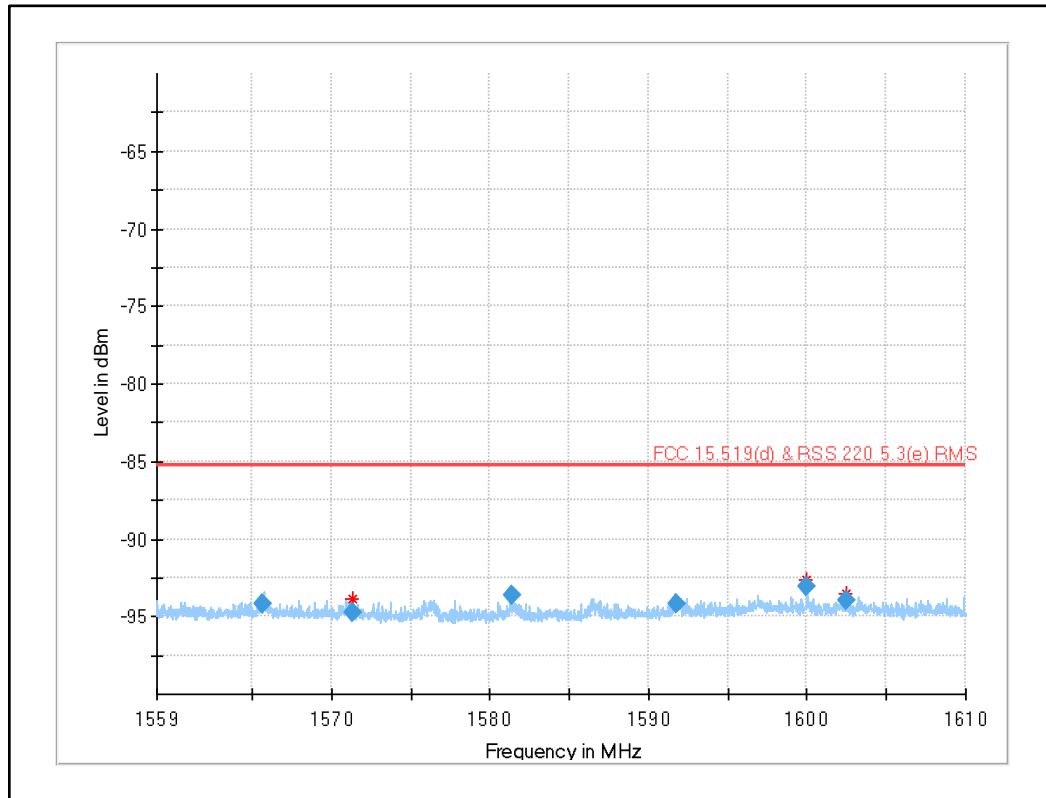
Plot 40: 1559 MHz to 1610 MHz (§15.519 (d), RSS-220 5.3.1(e)), UWB test mode channel 9 (SW version 02.11.13)
