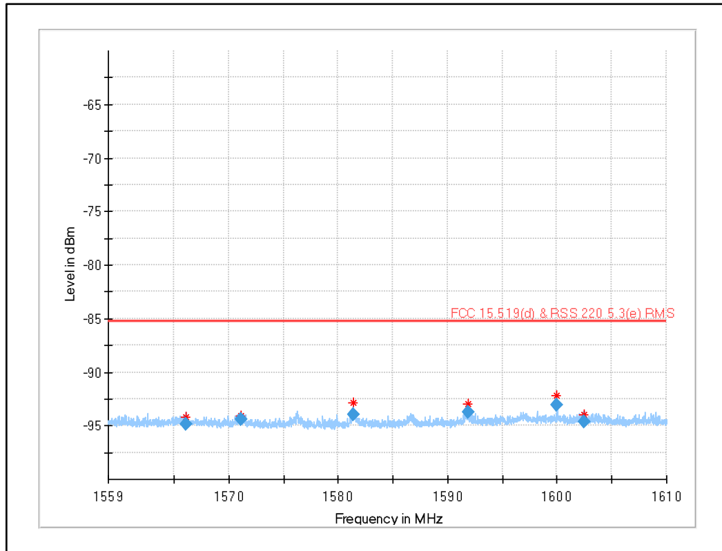
Plot 39: 1559 MHz to 1610 MHz (§15.519 (d), RSS-220 5.3.1(e)), UWB test mode channel 5 (SW version 02.11.13)
