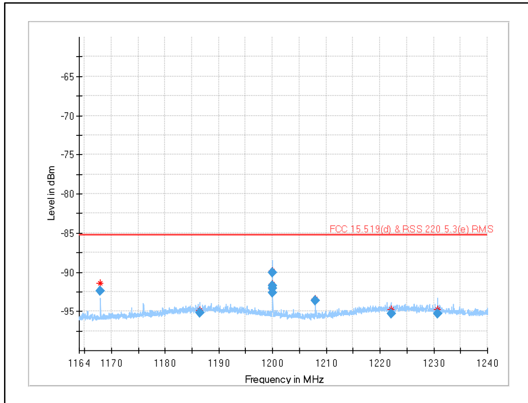
Plot 38: 1164 MHz to 1240 MHz (§15.519 (d), RSS-220 5.3.1(e)), UWB test mode channel 9 (SW version 02.11.13)
