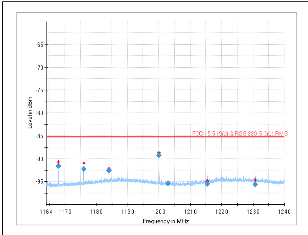
Plot 37: 1164 MHz to 1240 MHz (§15.519 (d), RSS-220 5.3.1(e)), UWB test mode channel 5 (SW version 02.11.13)
