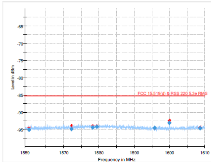
Plot 24: 1559 MHz to 1610 MHz (§15.519 (d), RSS-220 5.3.1(e)), CH 9
