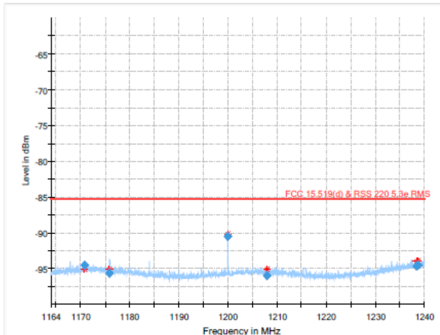
Plot 21: 1164 MHz to 1240 MHz (§15.519 (d), RSS-220 5.3.1(e)), CH 5
