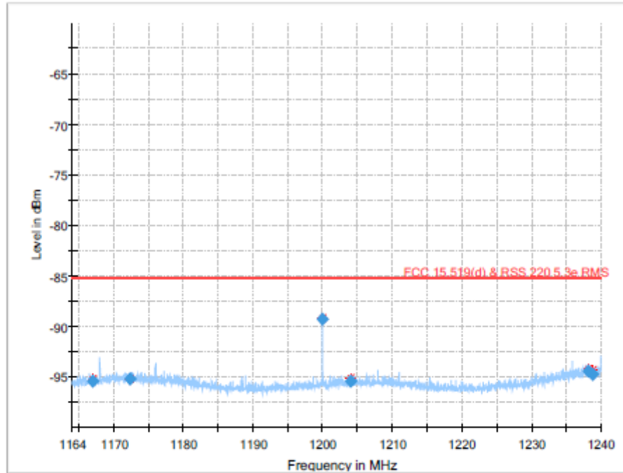
Plot 20: 1164 MHz to 1240 MHz (§15.519 (d), RSS-220 5.3.1(e)), CH 5
