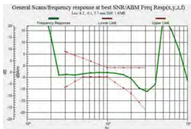
WCDMA850, Antenna 2
