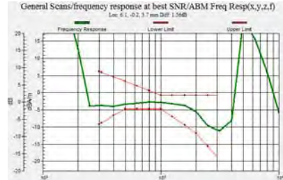
WCDMA1900, Antenna 2
