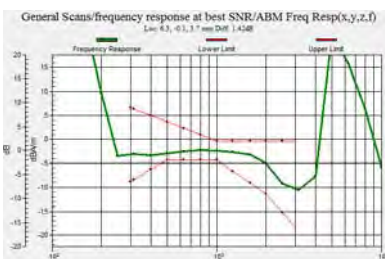
WCDMA1900, Antenna 1
