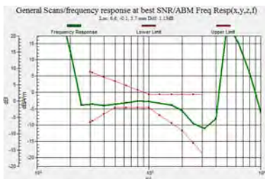
WCDMA1700/2100, Antenna 2
