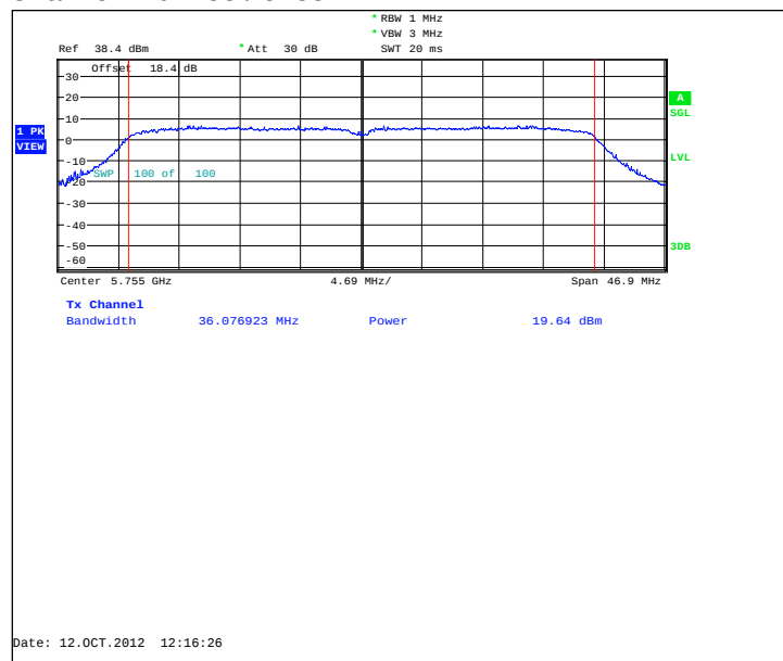
Channel 149+153 / 5755MHz
