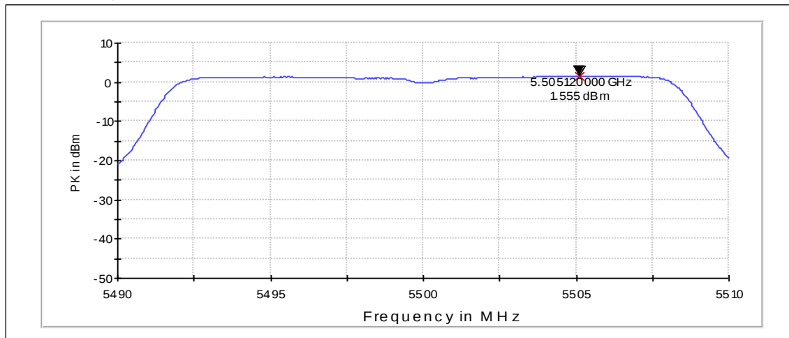
Channel 100 / 5500MHz
