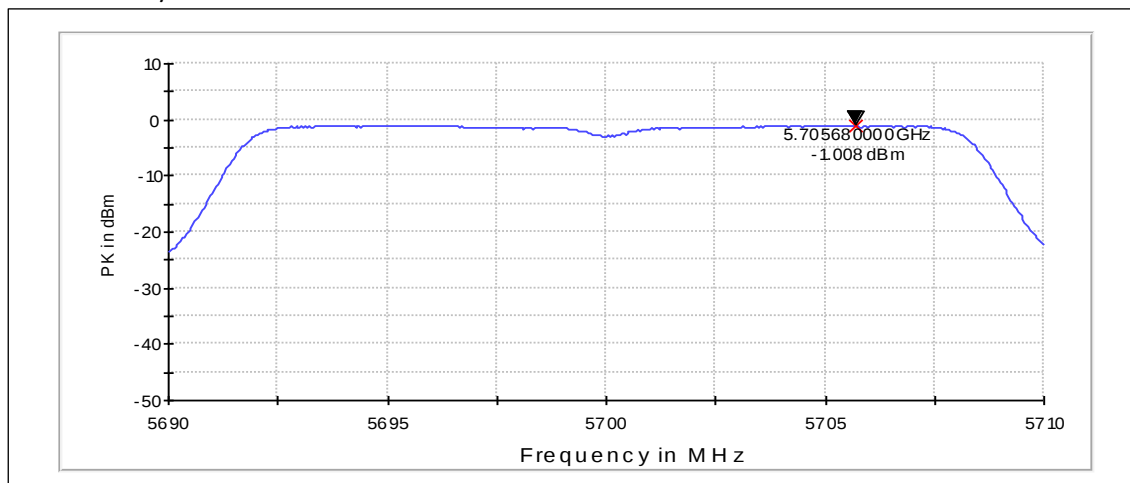
Channel 140 / 5700MHz
