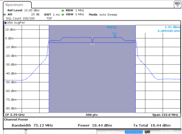
MIMO B-802.11ac-80MHz-Ch58-5290MHz-VHT0
