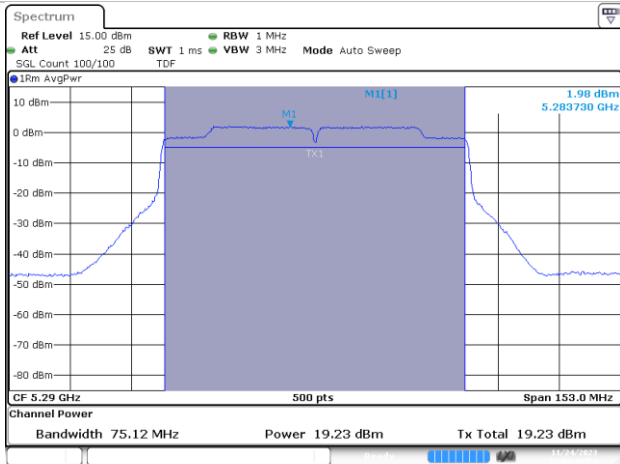
MIMO A-802.11ac-80MHz-Ch58-5290MHz-VHT0
