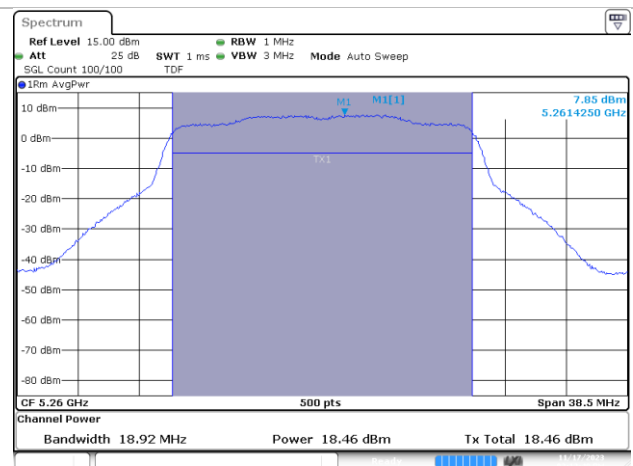
MIMO B-802.11ax/be-20MHz-Ch52-5260MHz-MCS0
