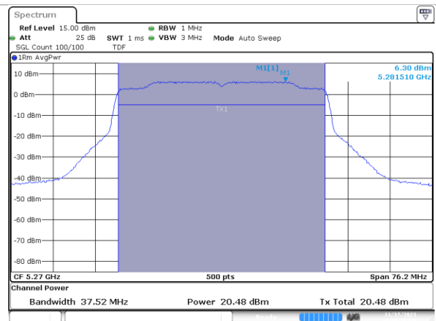
MIMO B-802.11ax/be-40MHz-Ch54-5270MHz-MCS0
