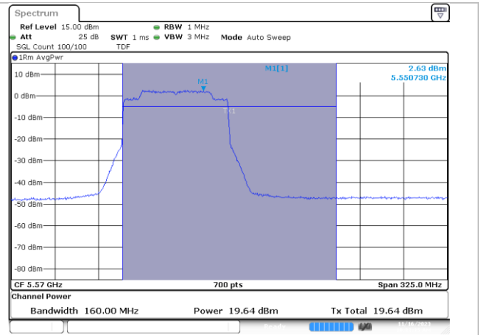
MIMO B-802.11ax/be160-Ch114-5570MHz-MCS0
