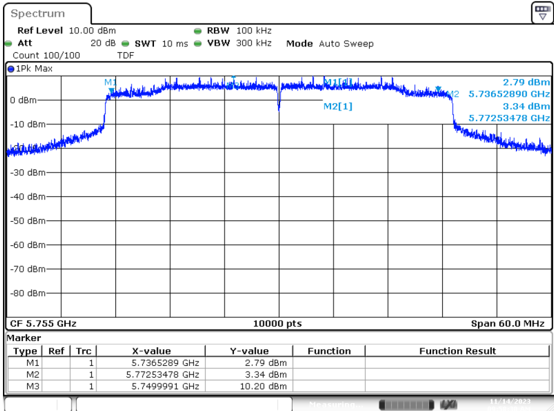
SISO B-802.11ax/be40-CH151-5755MHz-MCS0
