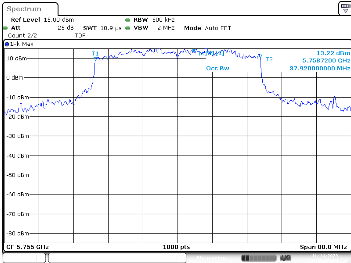
SISO B-802.11ax/be40-CH151-5755MHz-MCS0
