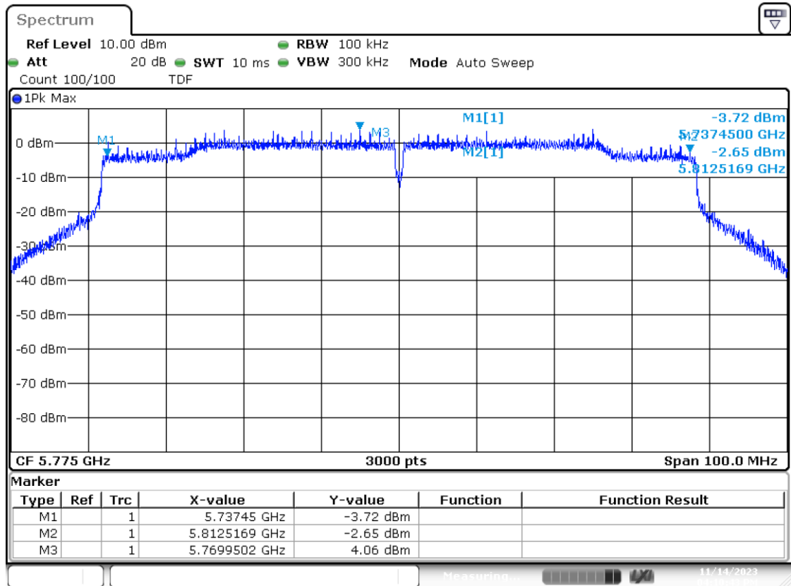
MIMO B-802.11ac80-CH155-5775MHz-VHT0
