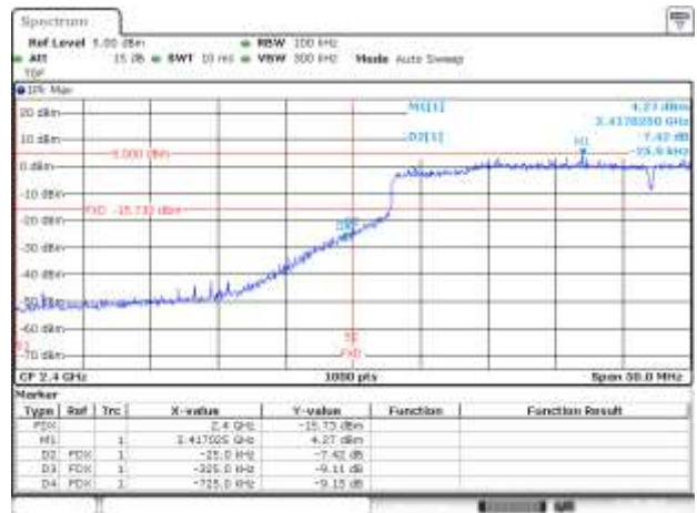
BE-NR, MIMO-A, 802.11ax40-MCS0, Ch3
