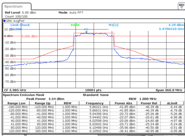
MIMO A-802.11ax/be-80MHz-Ch7-5985MHz-MCS0
