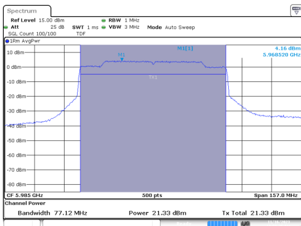
MIMO A-802.11ax/be-80MHz-Ch7-5985MHz-MCS0
