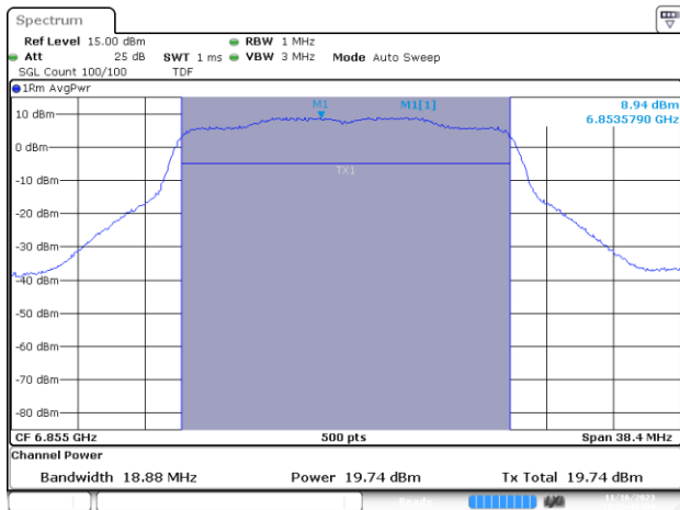
MIMO A-802.11ax/be-20MHz-Ch181-6855MHz-MCS0
