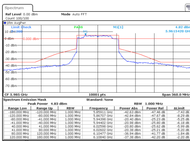
MIMO B-802.11ax/be-80MHz-Ch7-5985MHz-MCS0
