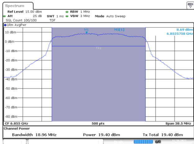
MIMO B-802.11ax/be-20MHz-Ch181-6855MHz-MCS0
