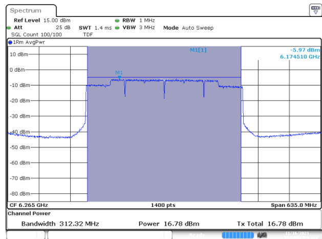
MIMO B-802.11be-320MHz-Ch63-6265MHz-MCS0
