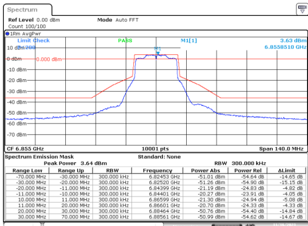
MIMO A-802.11ax/be-20MHz-Ch181-6855MHz-MCS0
