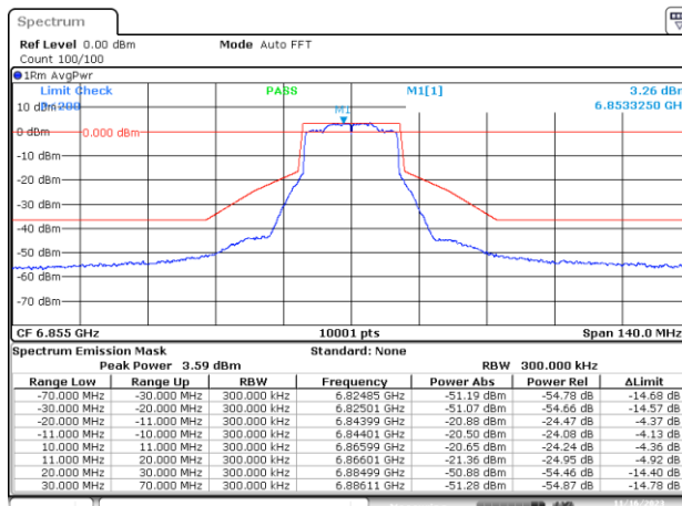
MIMO B-802.11ax/be-20MHz-Ch181-6855MHz-MCS0
