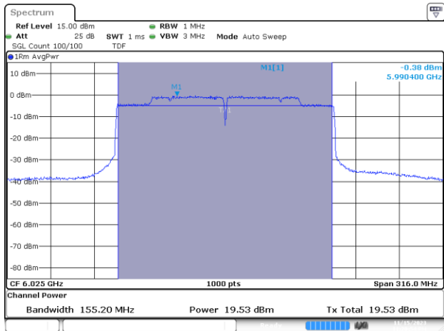
MIMO A-802.11ax/be-160MHz-Ch15-6025MHz-MCS0
