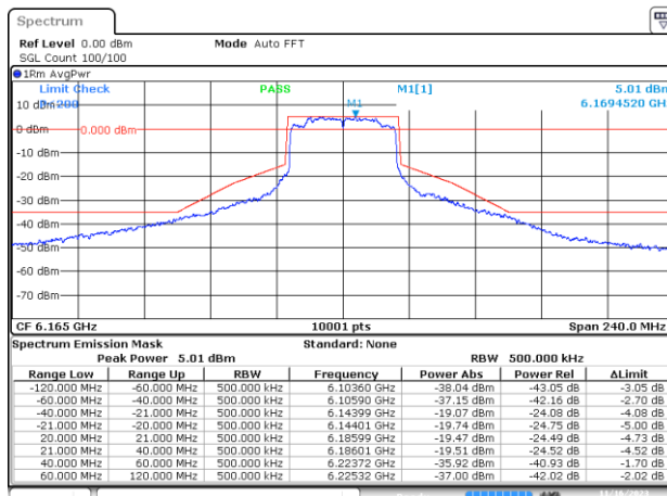
MIMO B-802.11ax/be-40MHz-Ch43-6165MHz-MCS0
