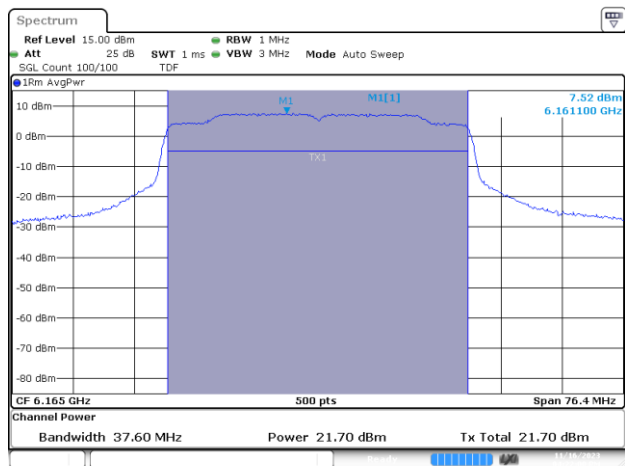
MIMO B-802.11ax/be-40MHz-Ch43-6165MHz-MCS0
