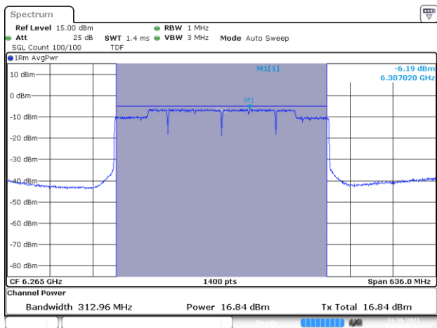
MIMO A-802.11be-320MHz-Ch63-6265MHz-MCS0
