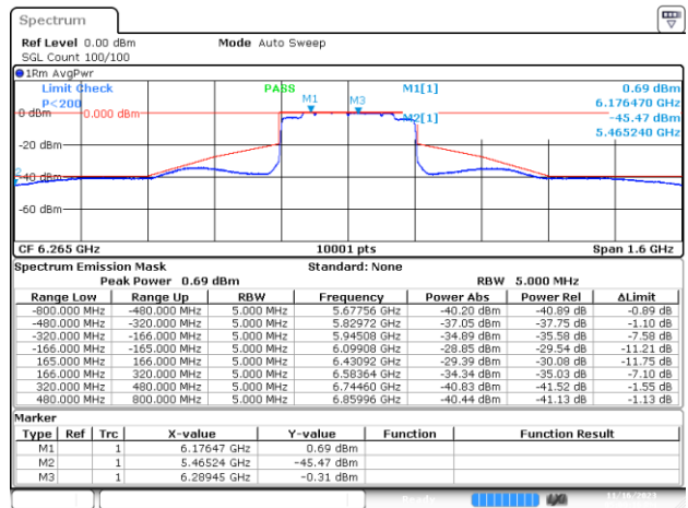
MIMO B-802.11be-320MHz-Ch63-6265MHz-MCS0
