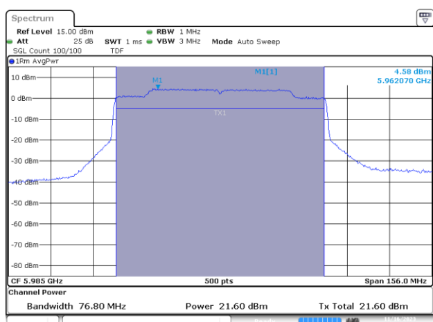
MIMO B-802.11ax/be-80MHz-Ch7-5985MHz-MCS0
