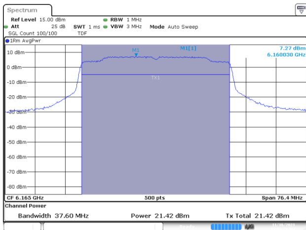
MIMO A-802.11ax/be-40MHz-Ch43-6165MHz-MCS0
