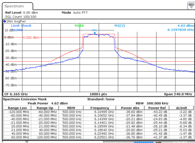
MIMO A-802.11ax/be-40MHz-Ch43-6165MHz-MCS0
