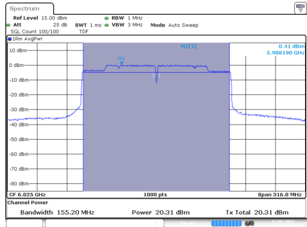
MIMO B-802.11ax/be-160MHz-Ch15-6025MHz-MCS0
