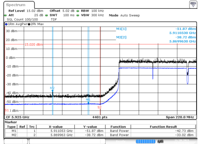
BE-NR-LOW, SISO-A, 802.11ax160-HE0, Ch15
