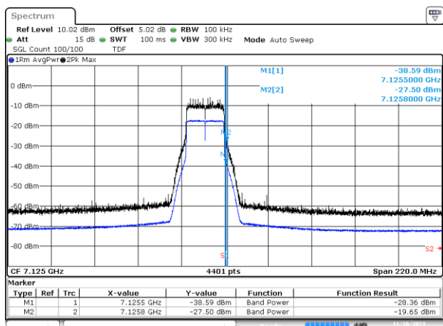
BE-NR-HIGH, SISO-A, 802.11ax20-HE0, Ch233
