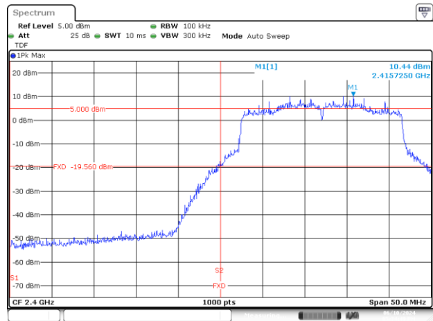
BE-NR, SISO-B, 802.11ax/be20-MCS0, Ch1
