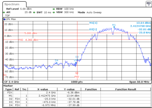
BE-NR, SISO-A, 802.11b-1Mbps, Ch1
