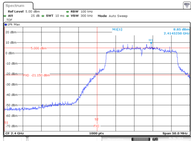
BE-NR, SISO-A, 802.11ax/be20-MCS0, Ch1
