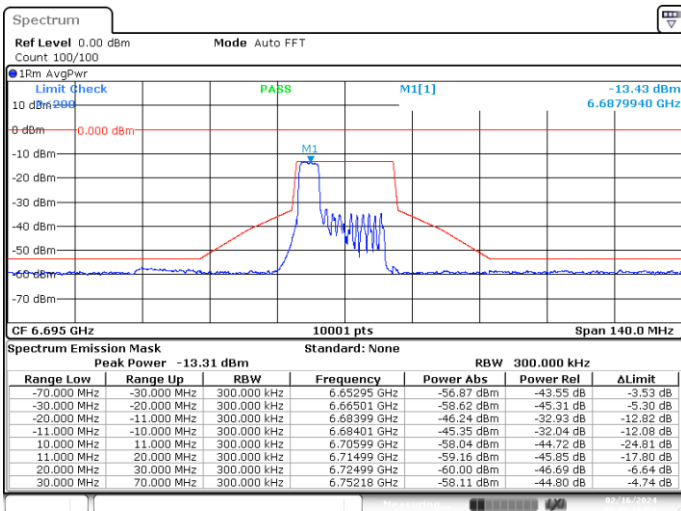
MIMO-A, 802.11ax/be20-MCS0, Ch149-3m-37
