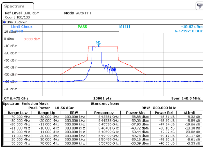
SISO-B, 802.11ax/be20-MCS0, Ch105-6m-70
