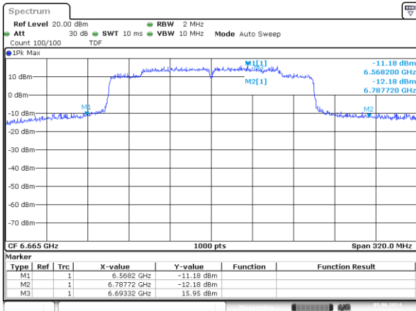
SISO-B 802.11ax/be160 ch143 26dB
