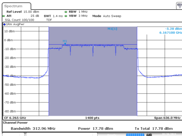
MIMO A-802.11be-320MHz-Ch63-MCS0
