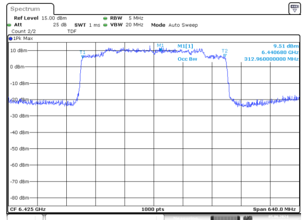
SISO-B 802.11be320 ch95 99%
