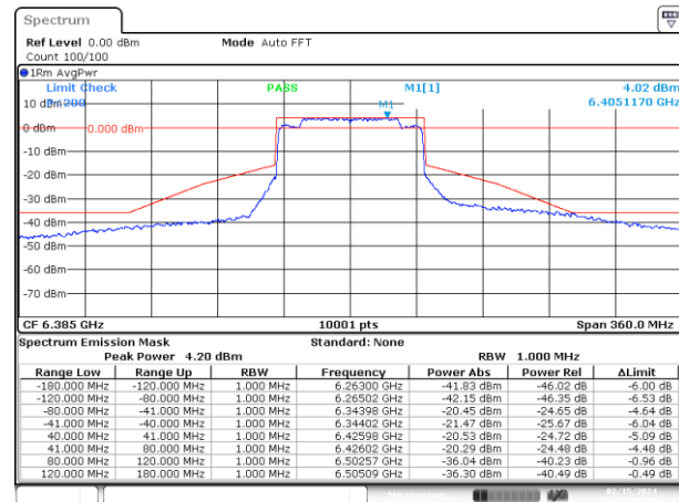
MIMO B-802.11ax/be-80MHz-Ch87-MCS0
