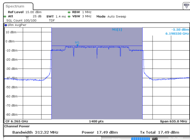
MIMO B-802.11be-320MHz-Ch63-MCS0
