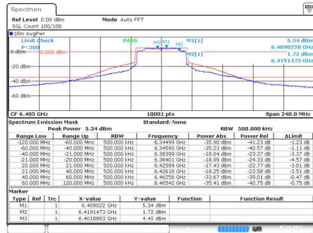
MIMO B-802.11ax/be-40MHz-Ch91-MCS0
