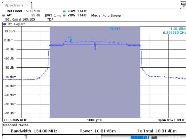
MIMO A-802.11ax/be-160MHz-Ch79-MCS0
