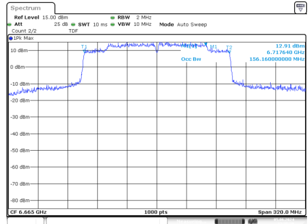
SISO-B 802.11ax/be160 ch143 99%
