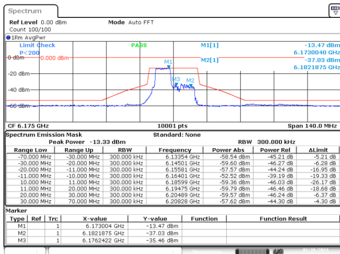
MIMO-A, 802.11ax/be20-MCS0, Ch45-6m-70
