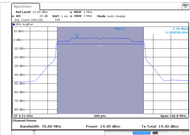
MIMO B-802.11ax/be-80MHz-Ch42-5210MHz-MCS0
