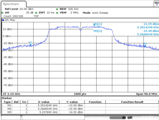
SISO A-802.11n-40MHz-46-5230-HT0-26dB
