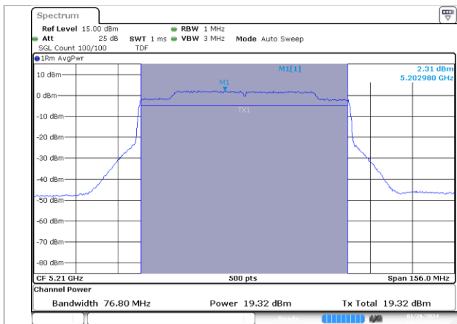
MIMO A-802.11ax/be-80MHz-Ch42-5210MHz-MCS0
