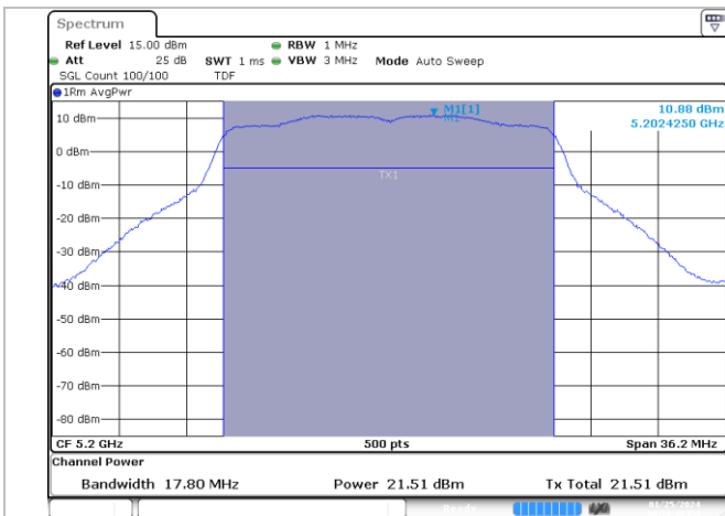
SISO B-802.11n-20MHz-Ch40-5200MHz-HT0
