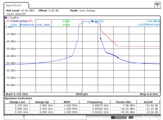
BE-NR-HIGH, MIMO-A, 802.11ax40-MCS0, Ch175
