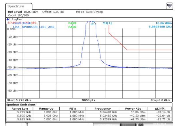
BE-NR-HIGH, SISO-B, 802.11a20-6Mbps, Ch173
