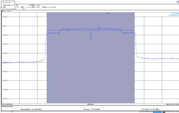
MIMO A-802.11ax-160MHz-Ch79-6345MHz-MCS0
