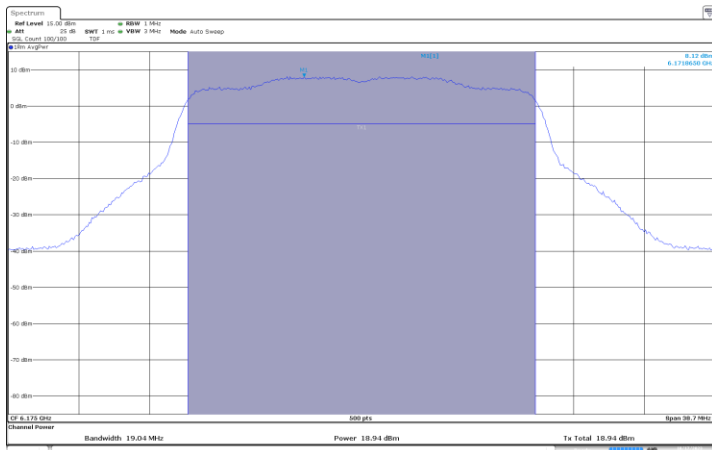
MIMO A-802.11ax-20MHz-Ch45-6175MHz-MCS0
