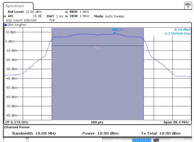
MIMO B-802.11ax-20MHz-Ch45-6175MHz-MCS0
