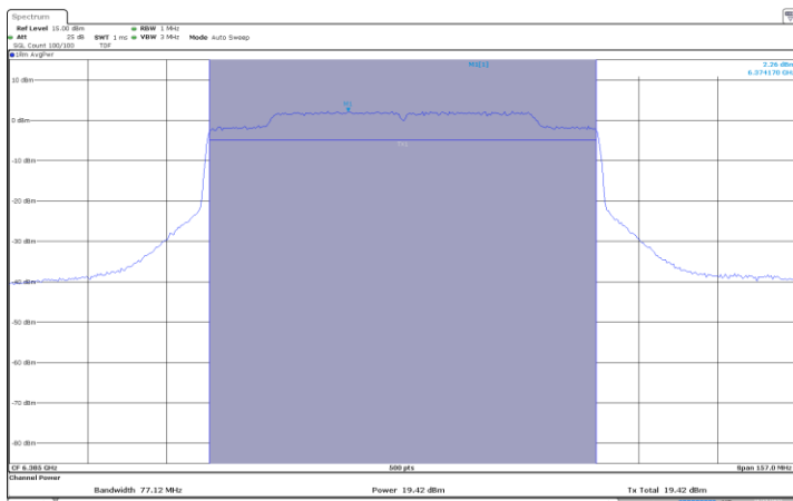
MIMO A-802.11ax-80MHz-Ch87-6385MHz-MCS0
