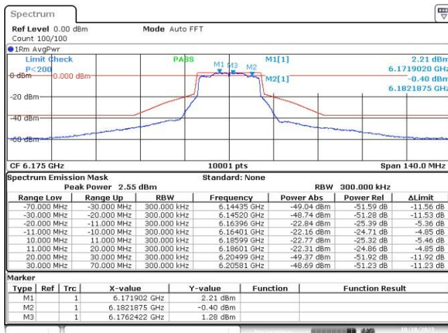
MIMO B-802.11ax-20MHz-Ch45-6175MHz-MCS0
