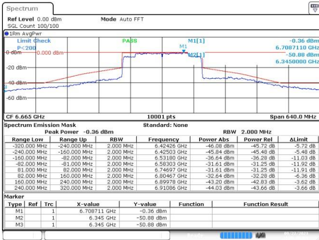
MIMO A-802.11ax-160MHz-Ch143-6665MHz-MCS0
