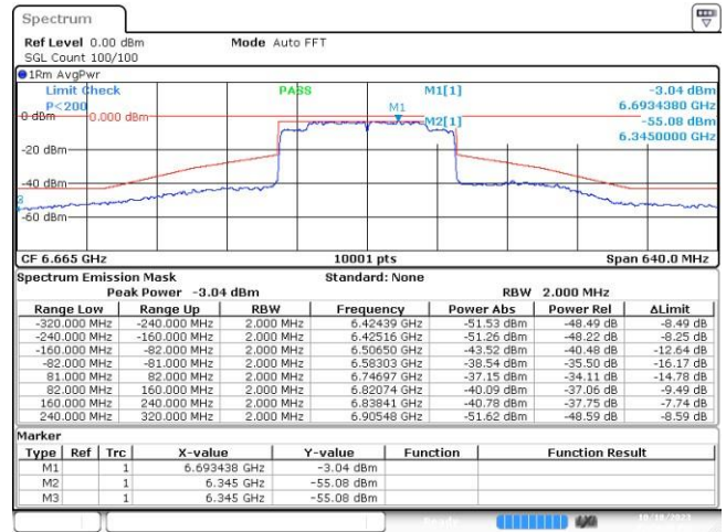
MIMO B-802.11ax-160MHz-Ch143-6665MHz-MCS0
