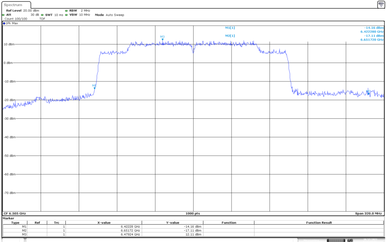
UNII-6 MIMO A 802.11ax160 CH111 6505MHz 26dB
