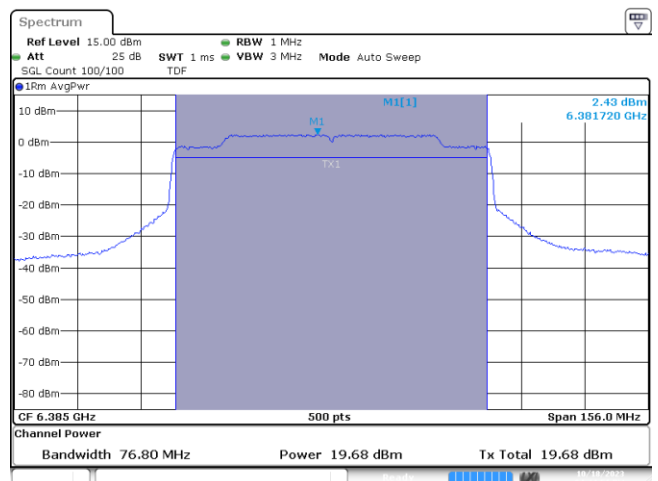
MIMO B-802.11ax-80MHz-Ch87-6385MHz-MCS0
