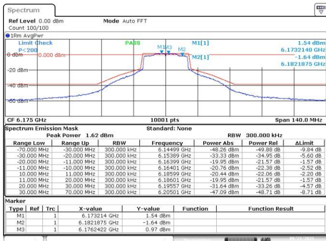
MIMO A-802.11ax-20MHz-Ch45-6175MHz-MCS0
