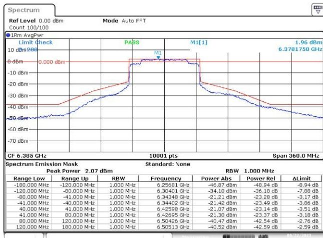
MIMO A-802.11ax-80MHz-Ch87-6385MHz-MCS0
