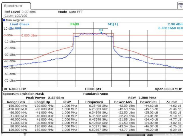
MIMO B-802.11ax-80MHz-Ch87-6385MHz-MCS0
