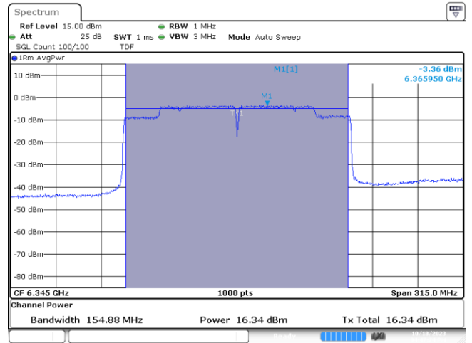
MIMO B-802.11ax-160MHz- Ch79-6345MHz-MCS0
