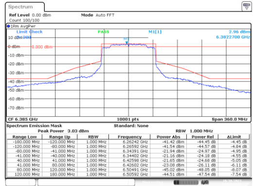
MIMO A-802.11ax-80MHz-Ch87-6385MHz-MCS0
