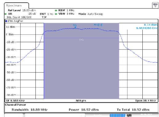
MIMO B-802.11ax-20MHz-Ch181-6855MHz-MCS0
