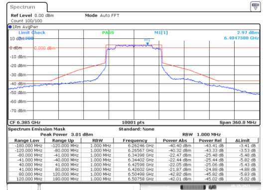
MIMO B-802.11ax-80MHz-Ch87-6385MHz-MCS0
