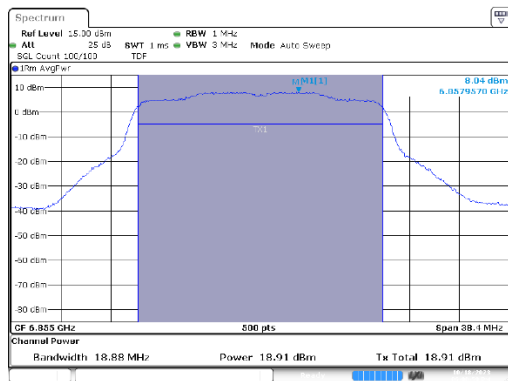
MIMO A-802.11ax-20MHz-Ch181-6855MHz-MCS0
