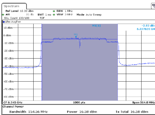
MIMO B-802.11ax-160MHz-Ch79-6345MHz-MCS0
