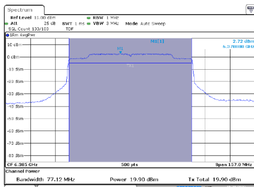
MIMO B-802.11ax-80MHz-Ch87-6385MHz-MCS0
