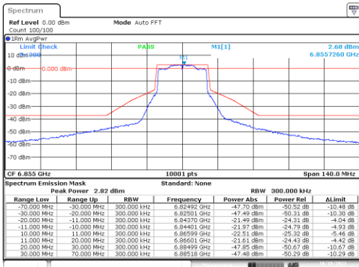
MIMO A-802.11ax-20MHz-Ch181-6855MHz-MCS0
