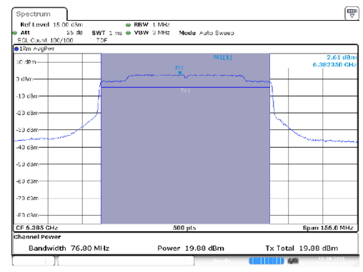
MIMO A-802.11ax-80MHz-Ch87-6385MHz-MCS0
