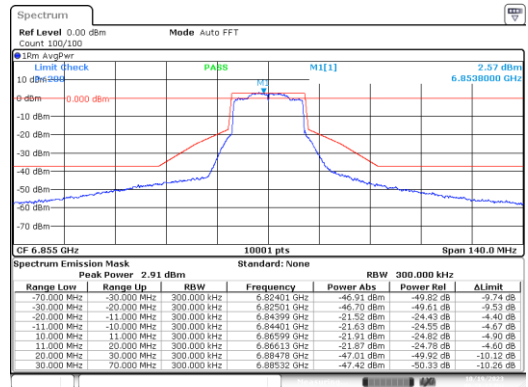
MIMO B-802.11ax-20MHz-Ch181-6855MHz-MCS0
