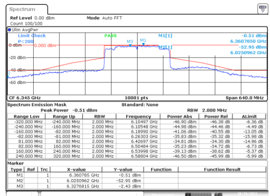
MIMO B-802.11ax-160MHz-Ch79-6345MHz-MCS0
