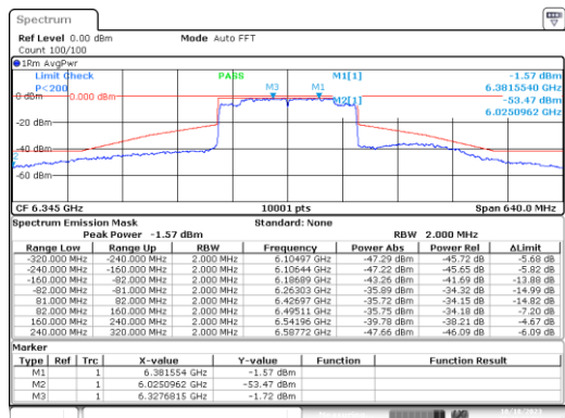
MIMO A-802.11ax-160MHz-Ch79-6345MHz-MCS0
