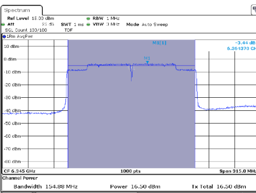
MIMO A-802.11ax-160MHz-Ch79-6345MHz-MCS0
