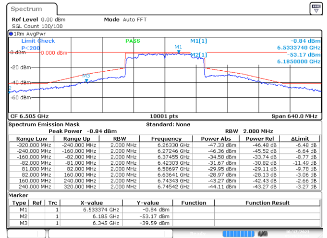
MIMO B-802.11ax-160MHz-Ch111-6505MHz-MCS0
