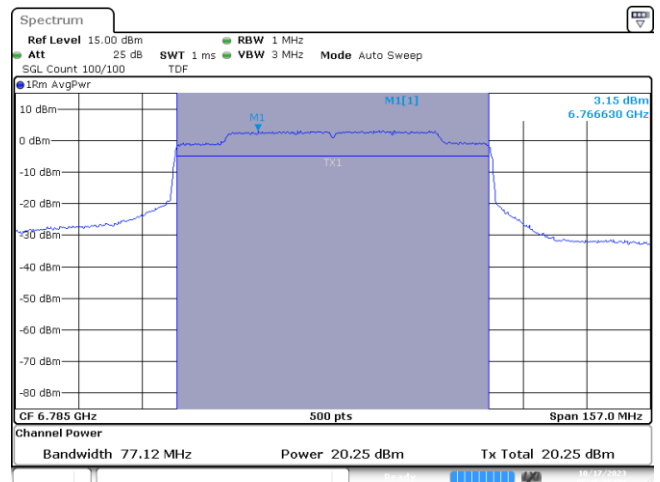
MIMO B-802.11ax-80MHz-Ch167-6785MHz-MCS0
