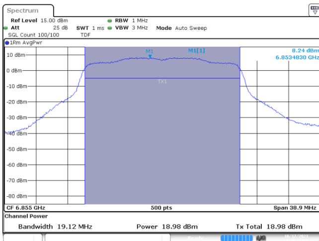
MIMO A-802.11ax-20MHz-Ch181-6855MHz-MCS0
