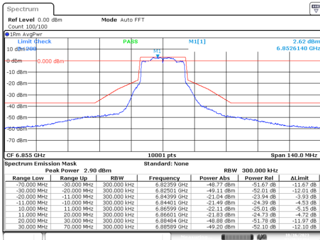
MIMO A-802.11ax-20MHz-Ch181-6855MHz-MCS0
