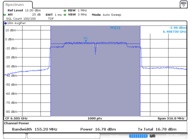
MIMO B-802.11ax-160MHz-Ch111-6505MHz-MCS0
