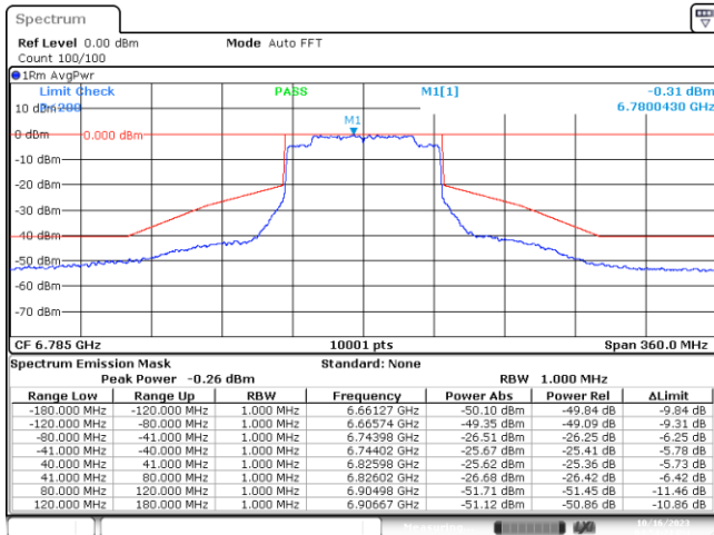
MIMO A-802.11ax-80MHz-Ch167-6785MHz-MCS0
