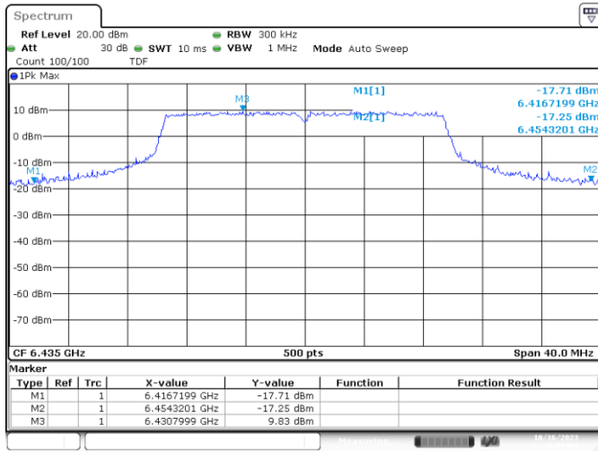
UNII-6 MIMO A 802.11ax20 CH97 6435MHz 26dB
