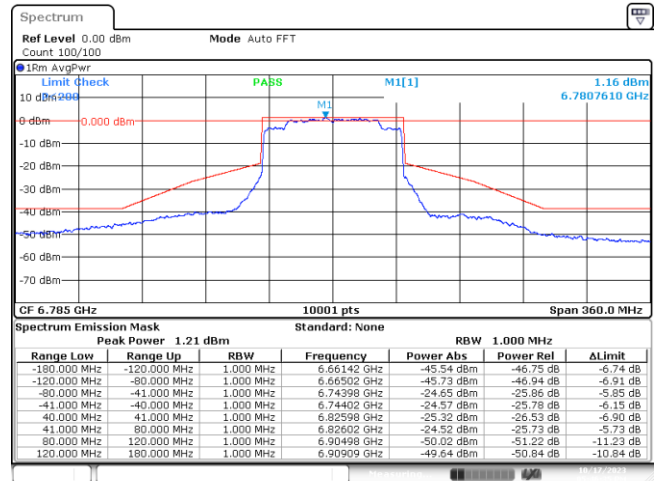
MIMO B-802.11ax-80MHz-Ch167-6785MHz-MCS0
