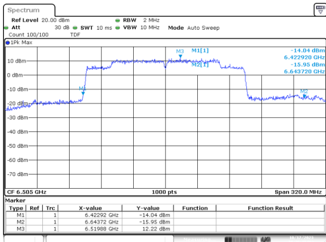
UNII-6 MIMO B 802.11ax160 CH111 6505MHz 26dB
