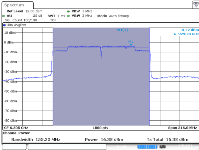
MIMO A-802.11ax-160MHz-Ch111-6505MHz-MCS0
