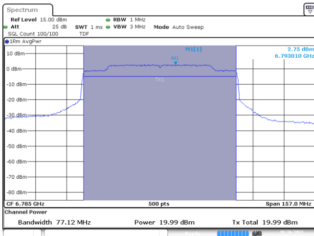
MIMO A-802.11ax-80MHz-Ch167-6785MHz-MCS0
