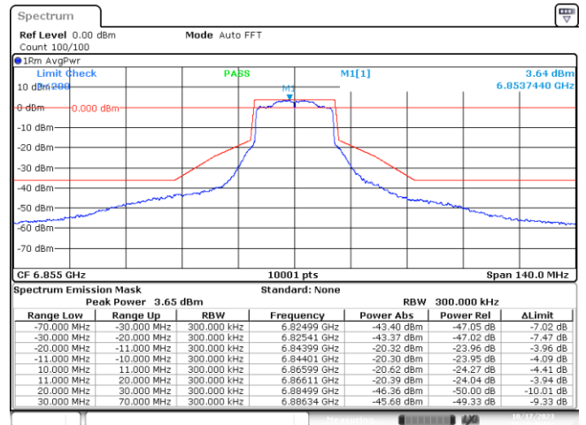
MIMO B-802.11ax-20MHz-Ch181-6855MHz-MCS0
