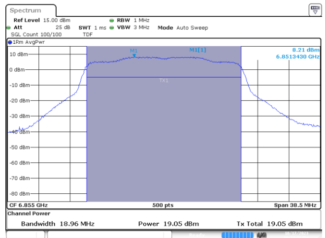
MIMO B-802.11ax-20MHz-Ch181-6855MHz-MCS0
