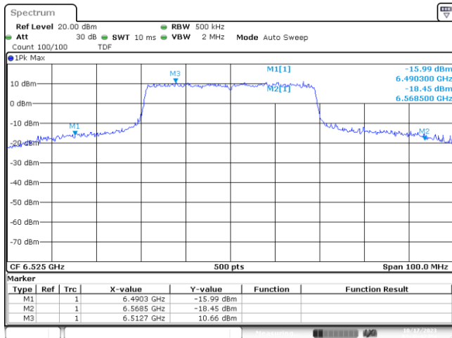
UNII-6 MIMO B 802.11ax40 CH115 6525MHz 26dB
