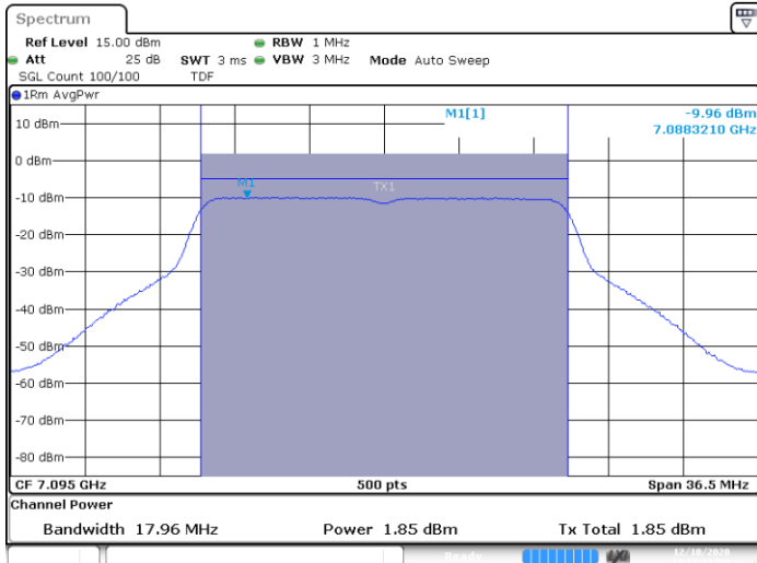
MIMO A-802.11n-20MHz-Ch229-7095MHz-HT8
