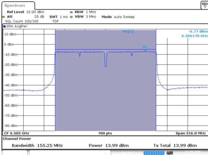
SISO A-802.11ac-160MHz-Ch111-6505MHz-VHT0
