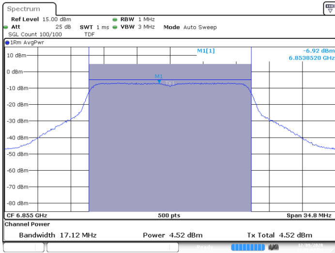
SISO A-802.11a-20MHz-Ch181-6855MHz-6
