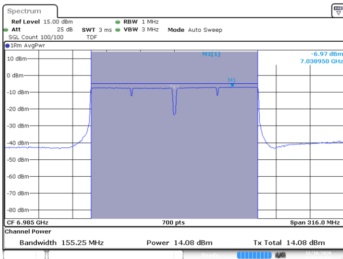
SISO A-802.11ac-160MHz-Ch207-6985MHz-VHT0
