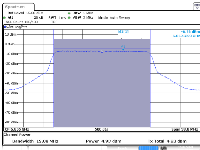
SISO B-802.11ax-20MHz-Ch181-6855MHz-HE0
