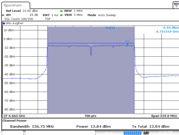
SISO A-802.11ax-160MHz-Ch143-6665MHz-HE0
