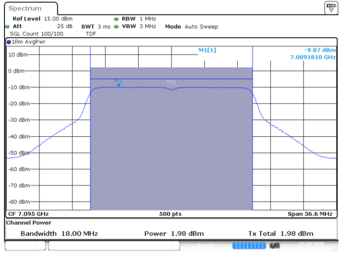
MIMO B-802.11n-20MHz-Ch229-7095MHz-HT8
