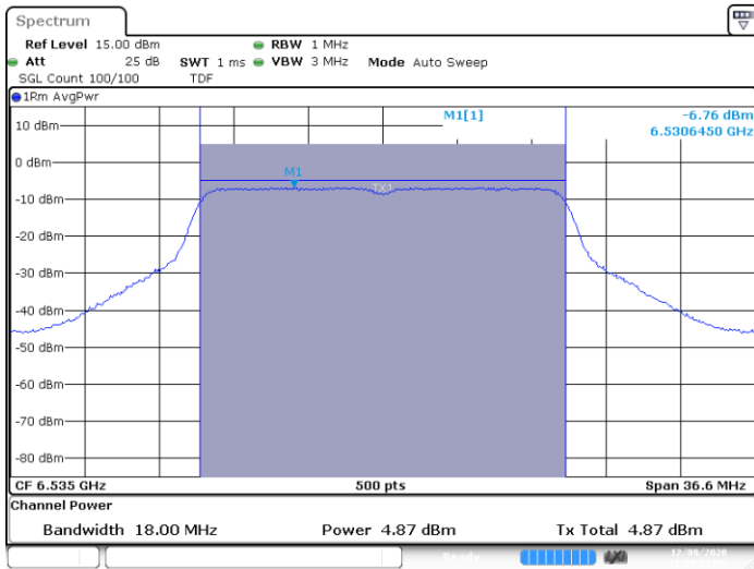
SISO A-802.11n-20MHz-Ch117-6535MHz-HT0
