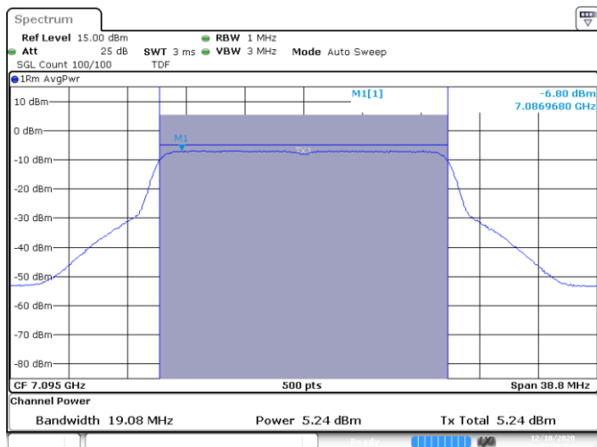
SISO B-802.11ax-20MHz-Ch229-7095MHz-HE0
