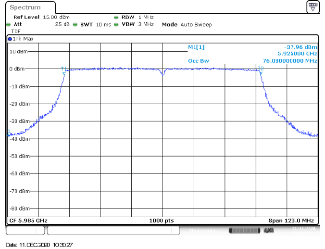
UNII5 MIMO A 802.11ac80 ch7 5985MHz 99%
