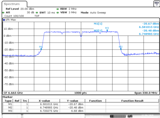
UNII7 SISO A 802.11ac160 ch143 6665MHz 26dB
