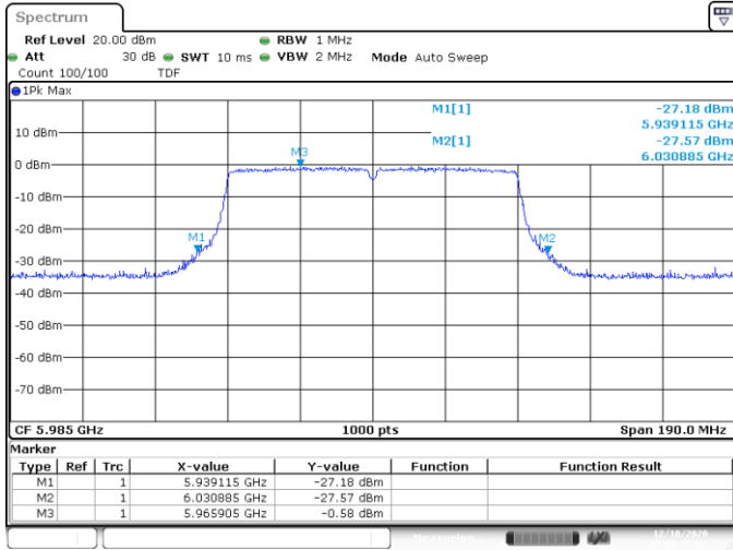
UNII5 MIMO A 802.11ac80 ch7 5985MHz 26dB
