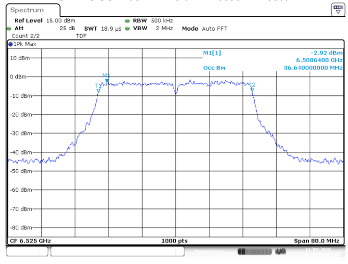
UNII7 SISO B 802.11n40 ch115 6525MHz 99%
