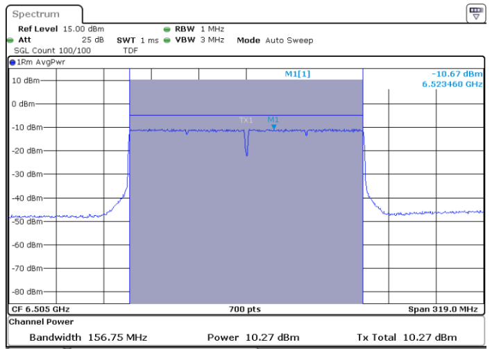
MIMO B-802.11ax-160MHz-Ch111-6505MHz-HE0
