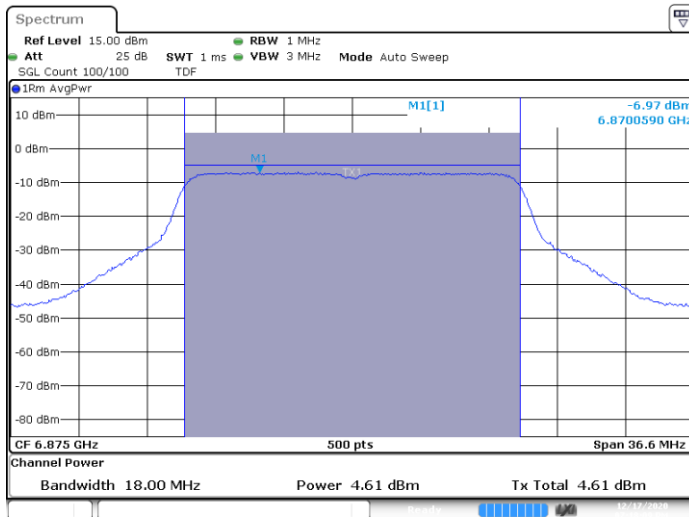
SISO B-802.11n-20MHz-Ch185-6875MHz-HT0
