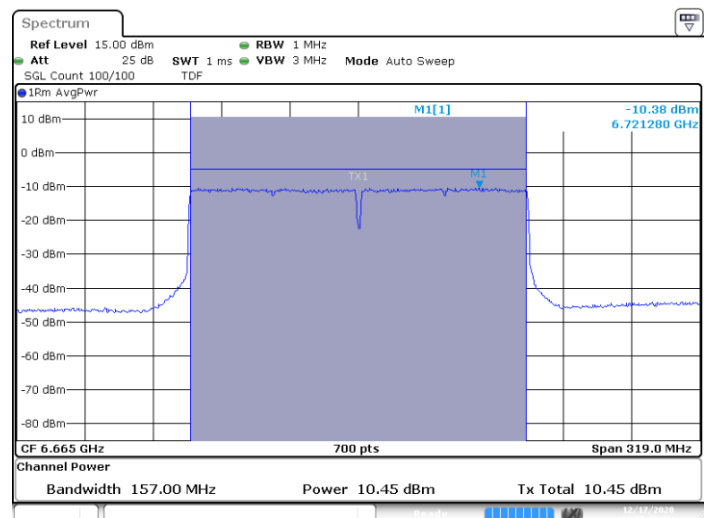
MIMO B-802.11ax-160MHz-Ch143-6665MHz-HE0
