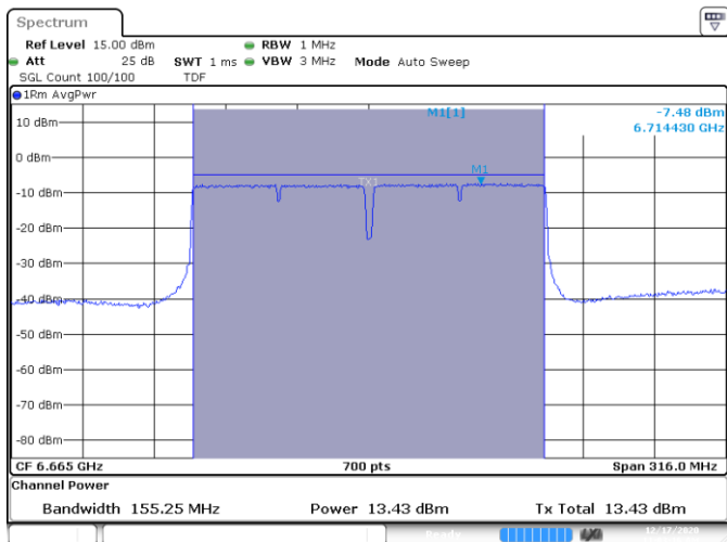
SISO A-802.11ac-160MHz-Ch143-6665MHz-VHT0
