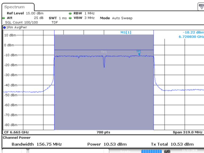
MIMO A-802.11ax-160MHz-Ch143-6665MHz-HE0
