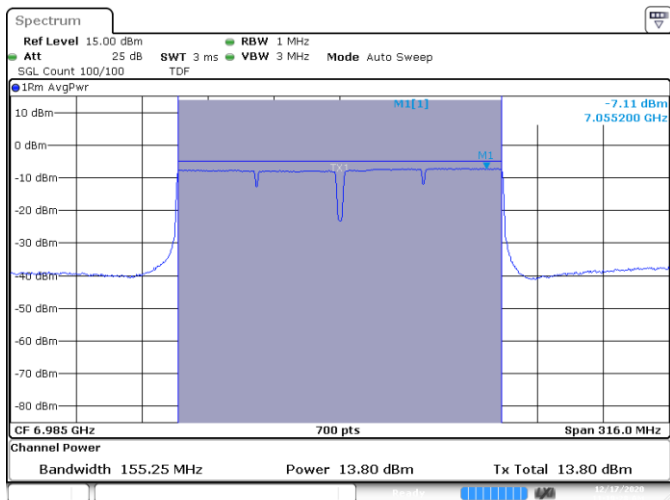
SISO A-802.11ac-160MHz-Ch207-6985MHz-VHT0
