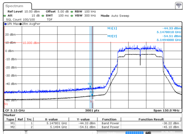
BE-R-LOW, MIMO-B, 802.11ax40-HE0, Ch38
