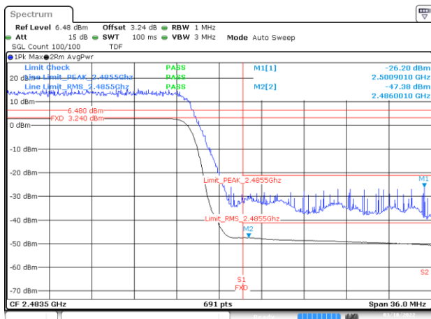
BE-R-HIGH, SISO-B, 802.11ax40-HE0, Ch11
