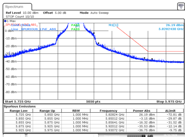
BE-NR-HIGH, SISO-B, 802.11ax20-HE0, Ch165
