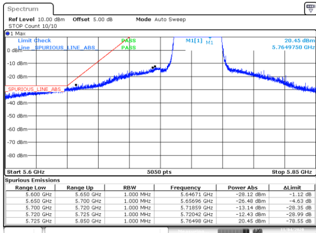
BE-NR-LOW, SISO-B, 802.11ax40-HE0, Ch151
