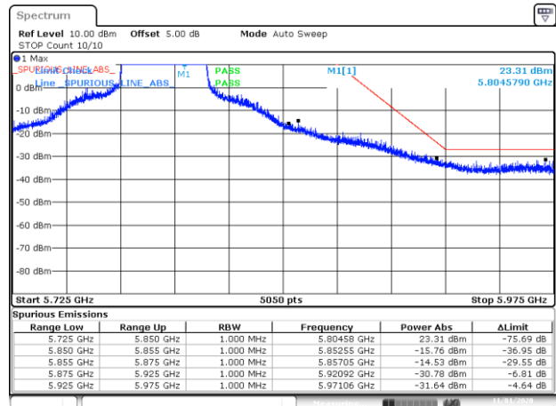
BE-NR-HIGH, SISO-B, 802.11ax40-HE0, Ch159
