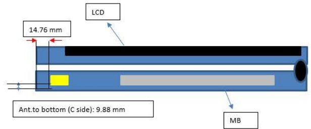
WLAN Aux/Tx2
