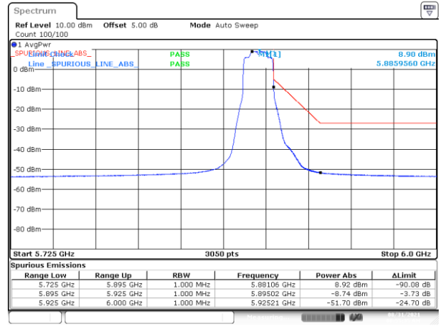
BE-NR-HIGH, MIMO-A, 802.11ax20-MCS0, Ch177
