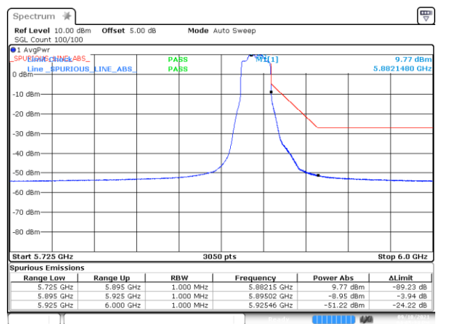
BE-NR-HIGH, MIMO-A, 802.11ax20-HE0, Ch177
