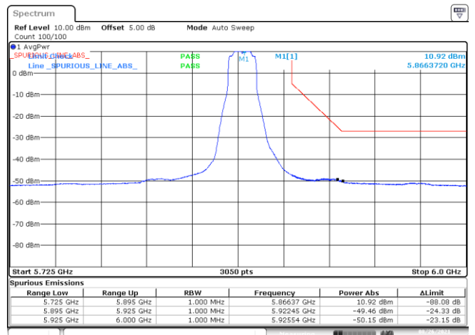
-BE-NR-HIGH, SISO-A, 802.11a20-6Mbps, Ch173
