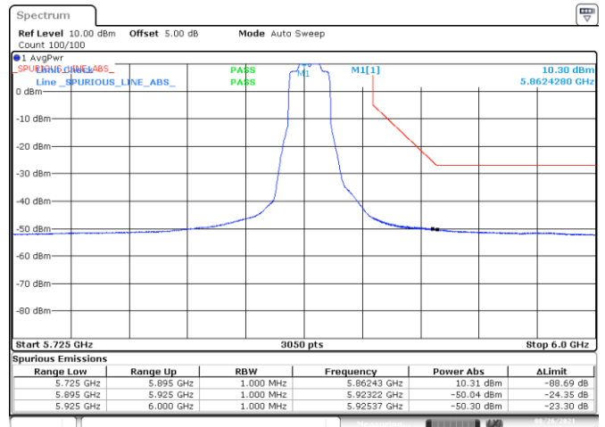
-BE-NR-HIGH, SISO-A, 802.11ax20-HE0, Ch173
