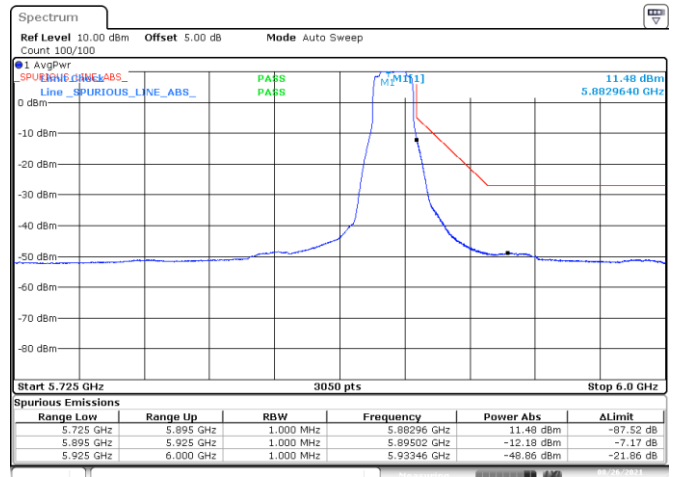
-BE-NR-HIGH, SISO-A, 802.11a20-6Mbps, Ch177
