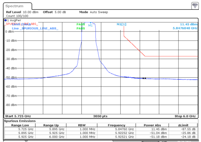
--BE-NR-HIGH, SISO-A, 802.11ax20-HE0, Ch169
