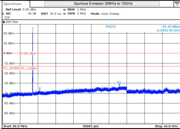
LTE 4 16QAM BW10MHz Mid Ch 20175 1RB-0
