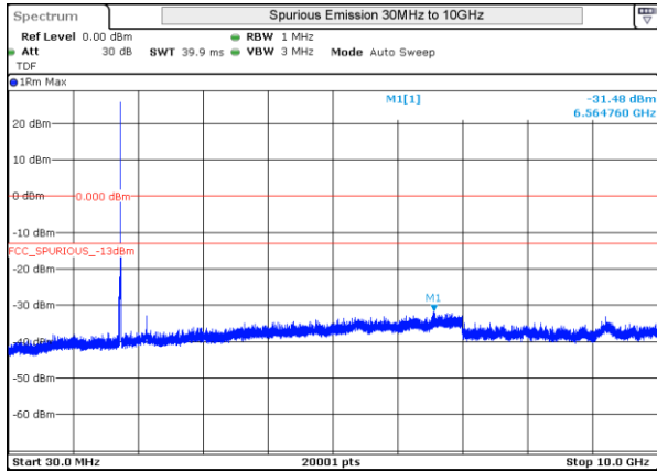
LTE 4 QPSK BW10MHz High Ch 20350 1RB-0
