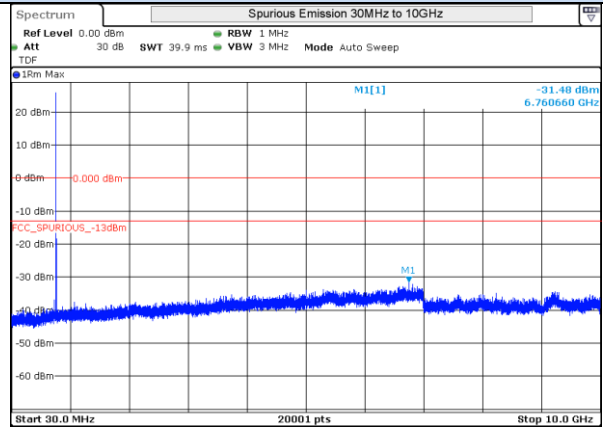
LTE 13 16QAM BW10MHz 782MHz High ch 23230 1RB-0
