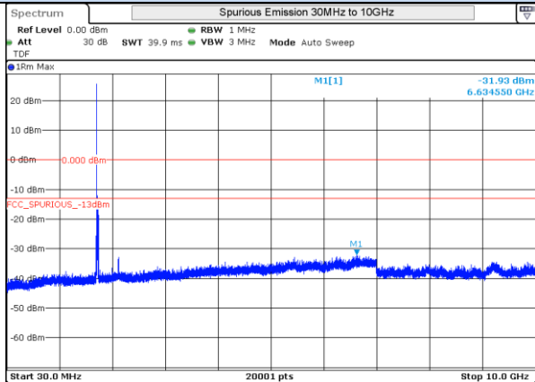
LTE 4 16QAM BW20MHz Mid Ch 20175 1RB-0
