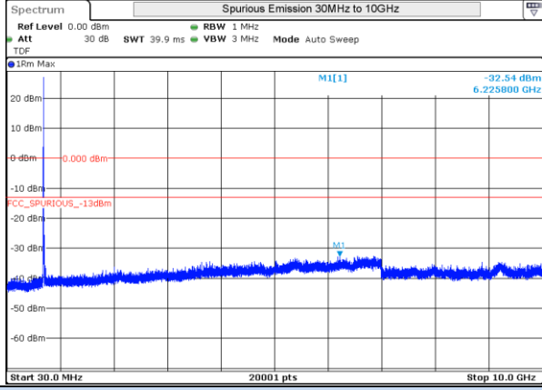
LTE 12 QPSK BW10MHz 704MHz Low ch 23060 1RB-0
