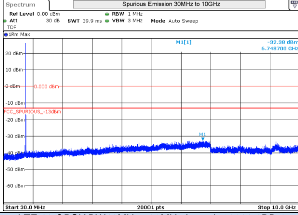
LTE 13 16QAM BW5MHz 782MHz Mid ch 23230 1RB-0
