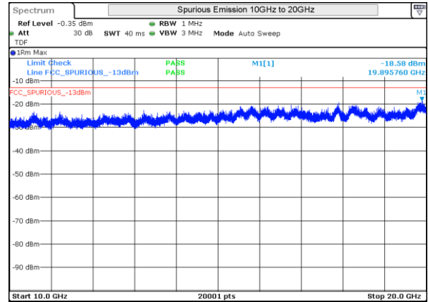
LTE 4 16QAM BW1.4MHz Mid Ch 20175 1RB-0
