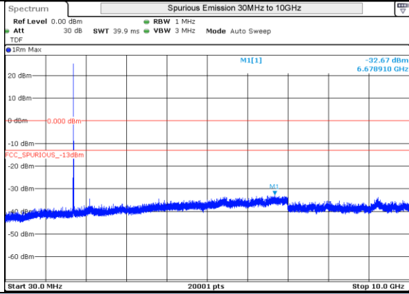
LTE 4 16QAM BW5MHz Low Ch 19975 1RB-0
