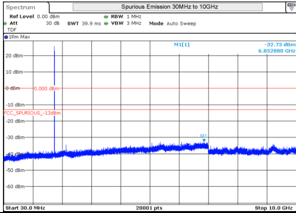
LTE 4 QPSK BW3MHz High Ch 20385 1RB-0
