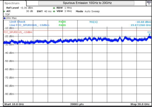
LTE 4 16QAM BW5MHz Low Ch 19975 1RB-0
