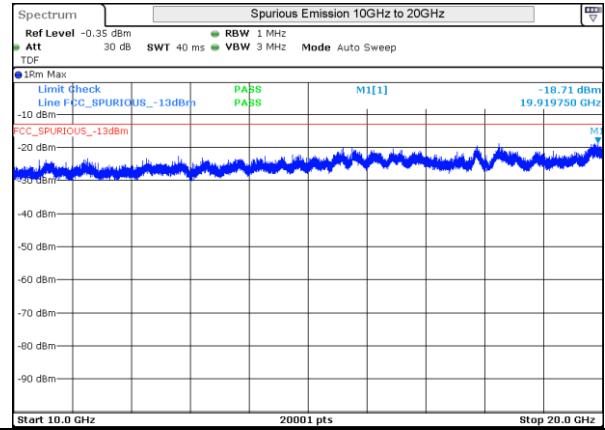
LTE 4 16QAM BW5MHz Mid Ch 20175 1RB-0
