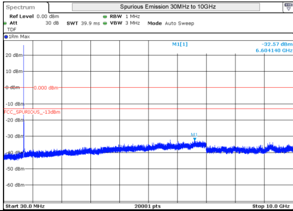
LTE 12 QPSK BW3MHz 714.5MHz High ch 23165 1RB-0
