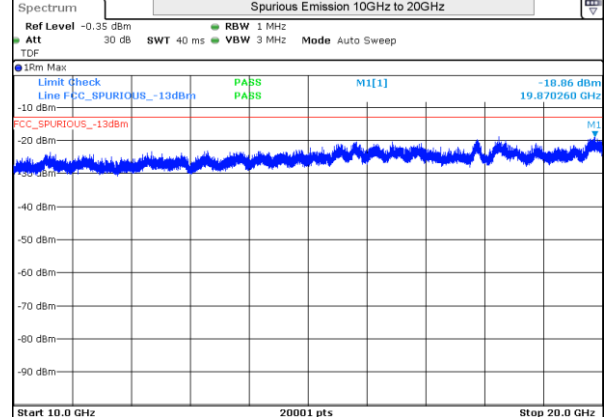
LTE 4 QPSK BW3MHz Low Ch 19965 1RB-0
