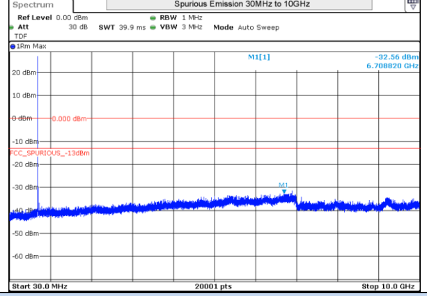
LTE 12 16QAM BW1.4MHz 707.5MHz Mid ch 23095 1RB-0
