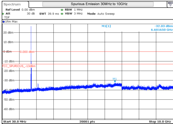
LTE 4 QPSK BW15MHz Low Ch 20025 1RB-0
