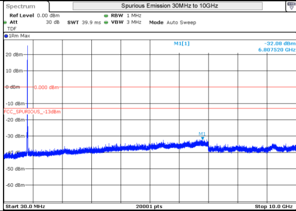
LTE 5 16QAM BW10MHz Mid Ch 20525 1RB-0
