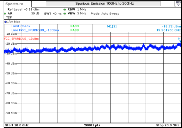
LTE 4 16QAM BW10MHz Mid Ch 20175 1RB-0
