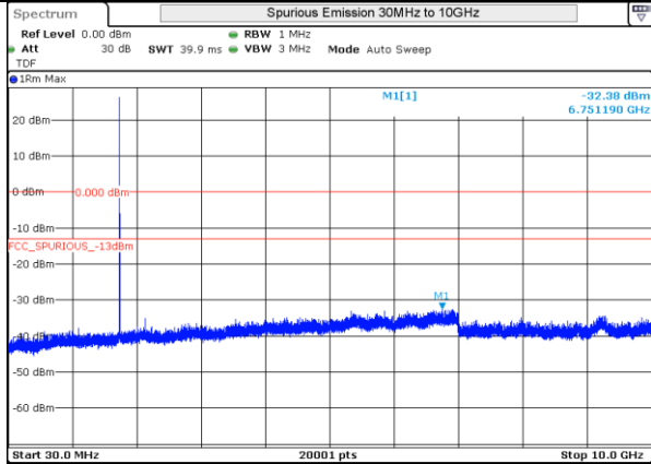
LTE 4 16QAM BW5MHz High Ch 20375 1RB-0
