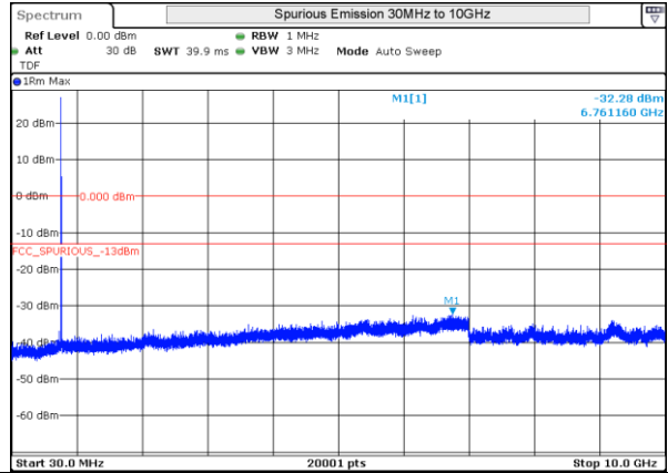
LTE 13 QPSK BW5MHz 782MHz Mid ch 23230 1RB-0
