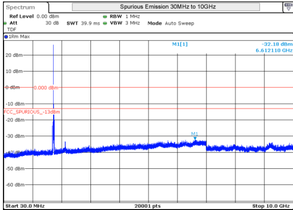
LTE 4 QPSK BW20MHz High Ch 20300 1RB-0
