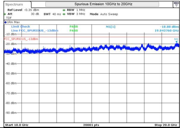
LTE 4 QPSK BW3MHz High Ch 20385 1RB-0
