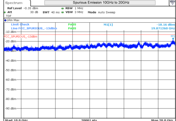
LTE 4 QPSK BW3MHz Mid Ch 20175 1RB-0
