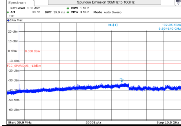
LTE 12 QPSK BW1.4MHz 715.3MHz High ch 23173 1RB-0
