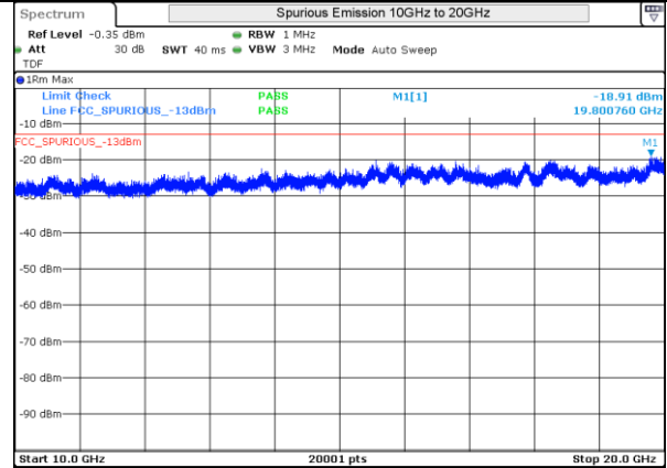
LTE 4 16QAM BW5MHz High Ch 20375 1RB-0
