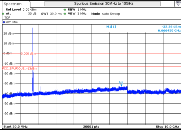
LTE 4 QPSK BW20MHz Mid Ch 20175 1RB-0
