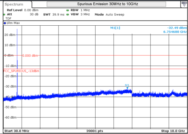
LTE 13 16QAM BW5MHz 779.5MHz Low ch 23205 1RB-0
