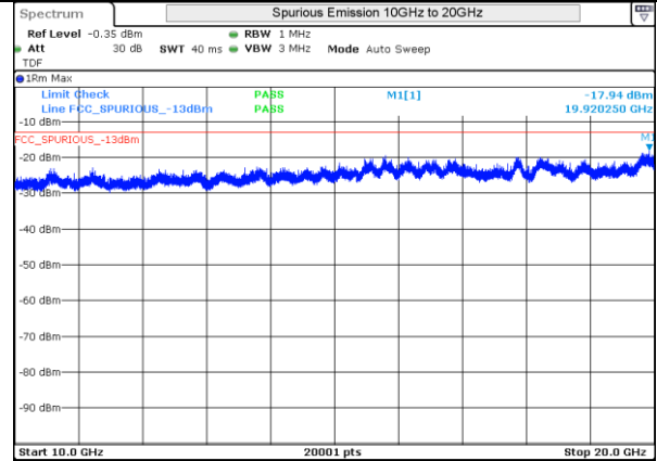
LTE 4 QPSK BW15MHz Mid Ch 20175 1RB-0
