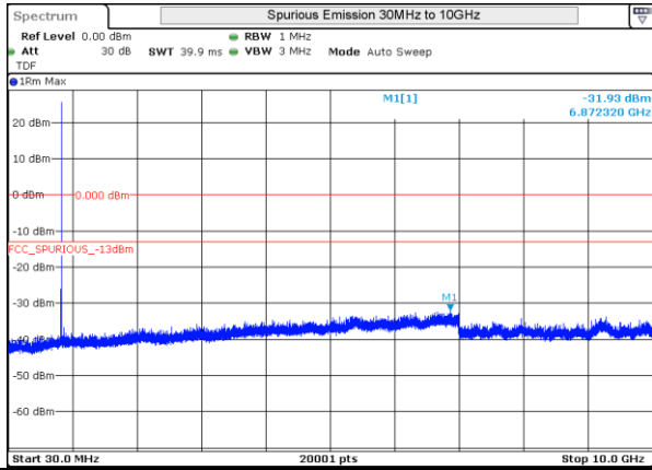
LTE 5 QPSK BW3MHz High Ch 20635 1RB-0
