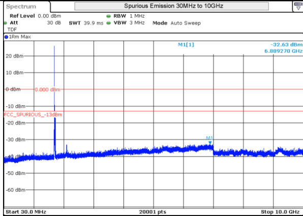
LTE 4 16QAM BW20MHz Low Ch 20050 1RB-0
