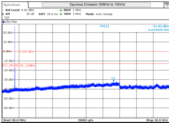
LTE 13 QPSK BW10MHz 782MHz High ch 23230 1RB-0
