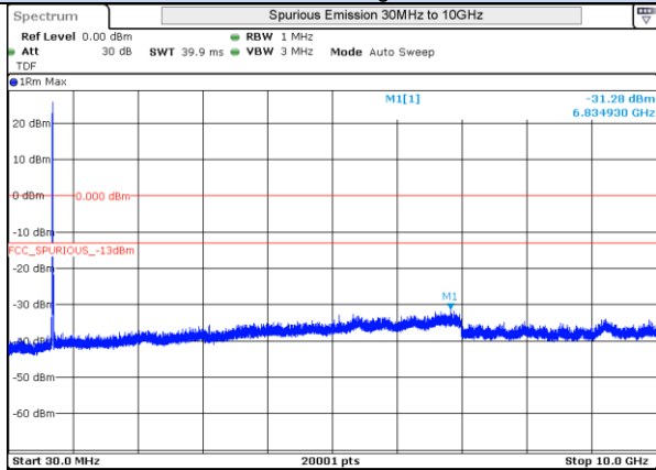
LTE 17 16QAM BW10MHz Mid Ch 23790 1RB-0
