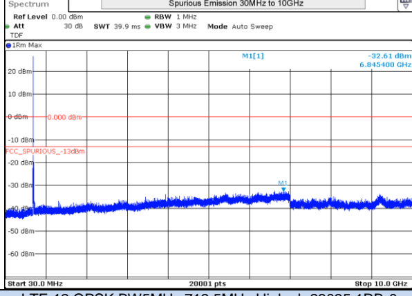
LTE 12 QPSK BW5MHz 713.5MHz High ch 23035 1RB-0
