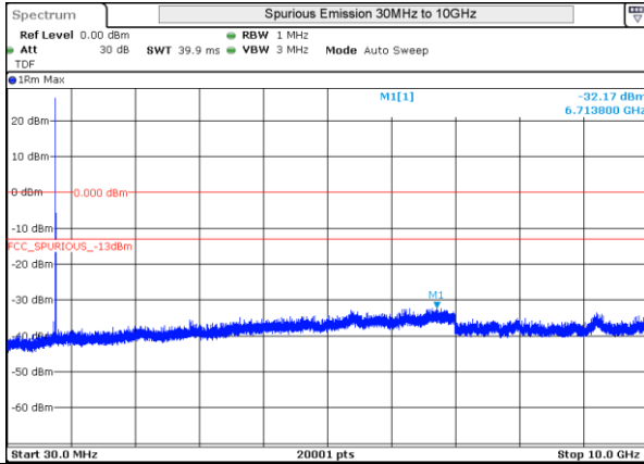
LTE 13 QPSK BW5MHz 779.5MHz Low ch 23205 1RB-0
