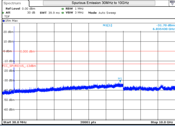
LTE 12 16QAM BW3MHz 707.5MHz Mid ch 23095 1RB-0
