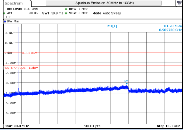
LTE 5 QPSK BW5MHz Mid Ch 20525 1RB-0
