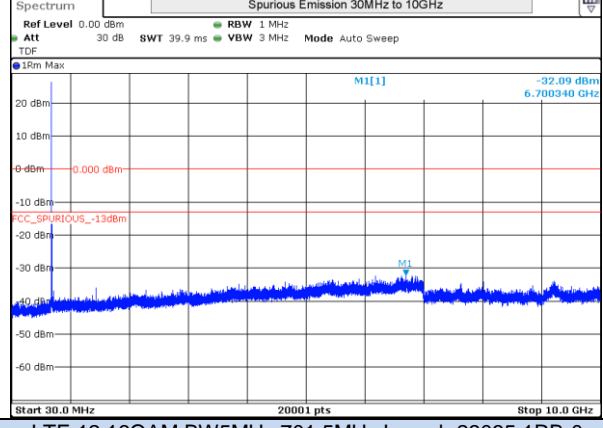
LTE 12 16QAM BW5MHz 701.5MHz Low ch 23035 1RB-0
