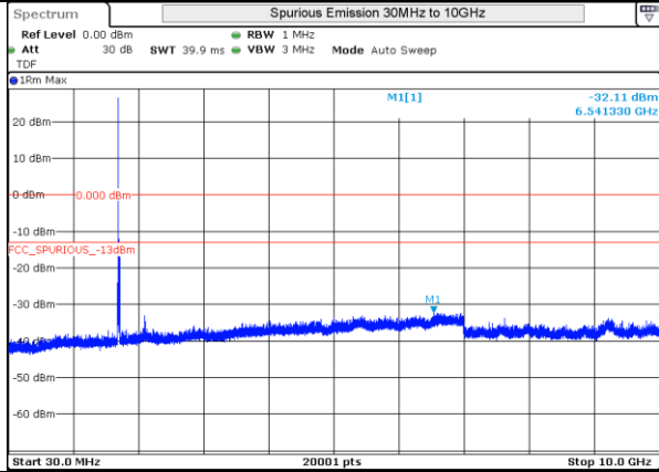
LTE 4 QPSK BW10MHz Low Ch 20000 1RB-0
