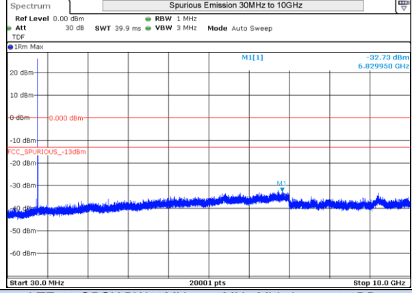
LTE 13 16QAM BW5MHz 784.5MHz High ch 23255 1RB-0
