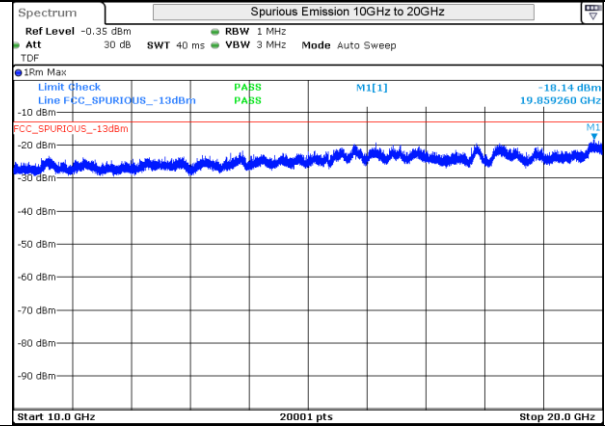
LTE 4 16QAM BW10MHz High Ch 20350 1RB-0
