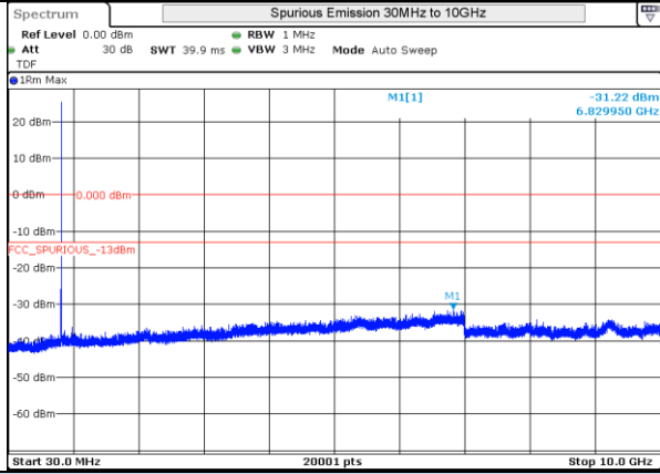
LTE 5 16QAM BW3MHz Mid Ch 20525 1RB-0
