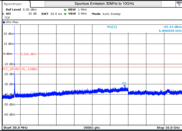
LTE 12 16QAM BW5MHz 707.5MHz Mid ch 23095 1RB-0
