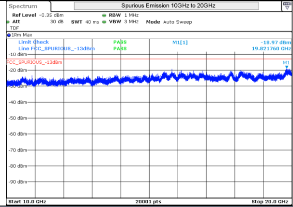
LTE 4 QPSK BW20MHz Mid Ch 20175 1RB-0
