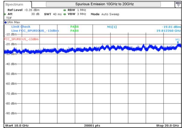
LTE 4 QPSK BW10MHz High Ch 20350 1RB-0
