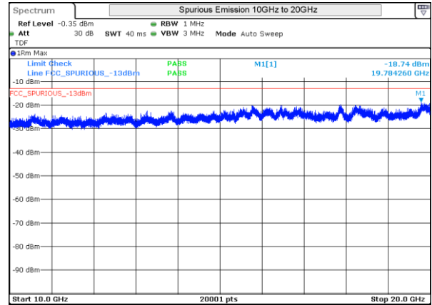
LTE 4 QPSK BW15MHz Low Ch 20025 1RB-0
