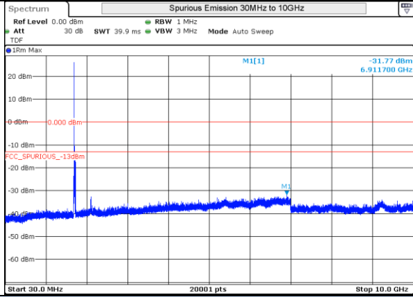
LTE 4 QPSK BW20MHz Low Ch 20050 1RB-0
