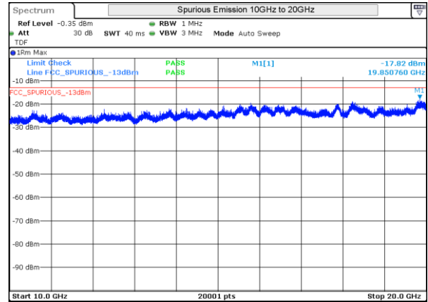
LTE 4 QPSK BW20MHz High Ch 20300 1RB-0
