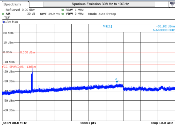
LTE 4 16QAM BW20MHz High Ch 20300 1RB-0
