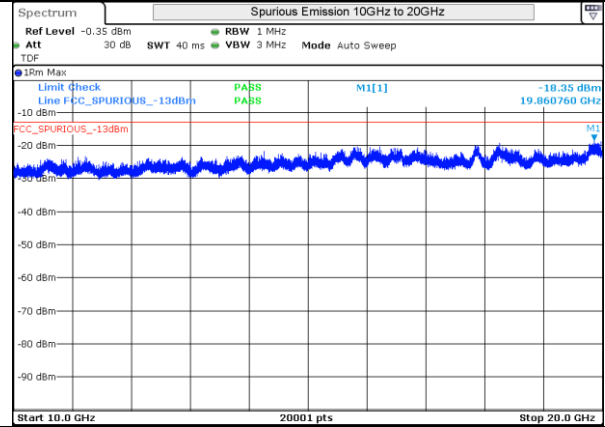
LTE 4 QPSK BW10MHz Low Ch 20000 1RB-0
