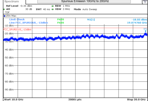
LTE 4 16QAM BW1.4MHz High Ch 20393 1RB-0
