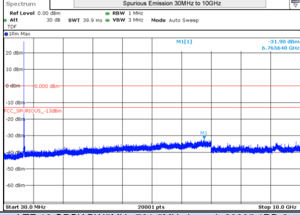
LTE 12 QPSK BW5MHz 701.5MHz Low ch 23035 1RB-0
