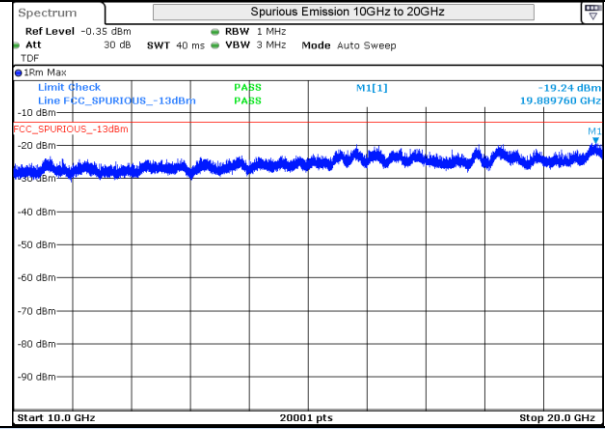
LTE 4 QPSK BW5MHz High Ch 20375 1RB-0
