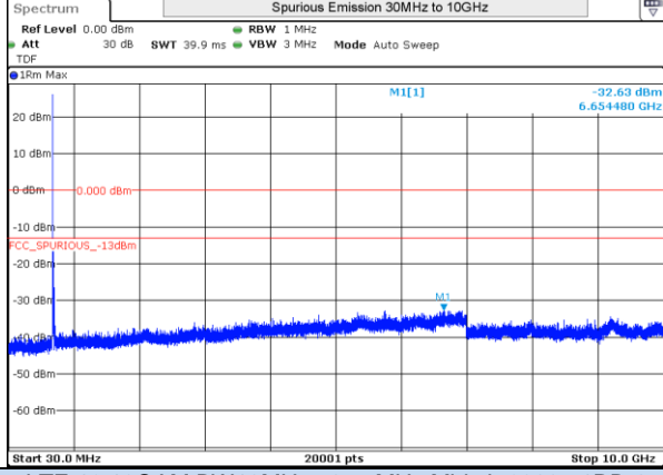
LTE 12 QPSK BW10MHz 711MHz High ch 23130 1RB-0
