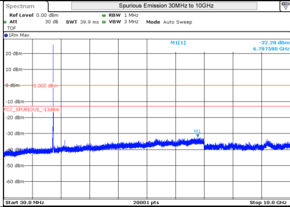
LTE 4 16QAM BW10MHz High Ch 20350 1RB-0
