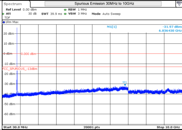
LTE 5 QPSK BW10MHz High Ch 20600 1RB-0
