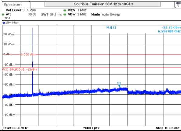
LTE 4 QPSK BW5MHz Low Ch 19975 1RB-0
