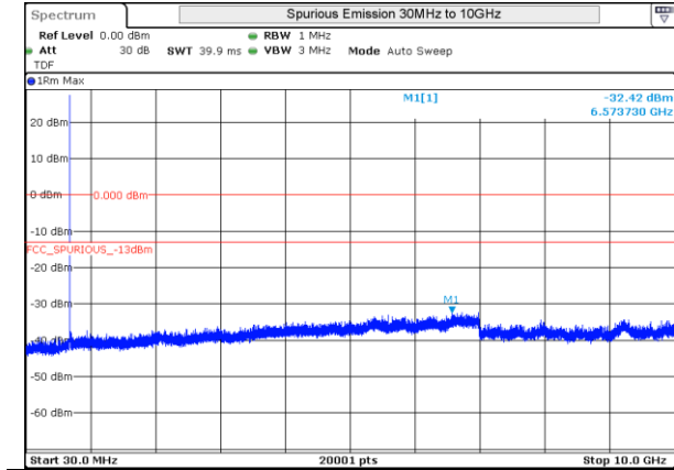
LTE 12 QPSK BW1.4MHz 699.7MHz Low ch 23017 1RB-0
