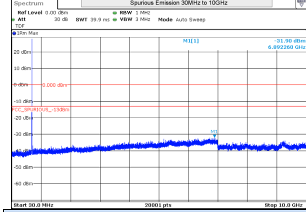
LTE 12 16QAM BW1.4MHz 715.3MHz High ch 23173 1RB-0
