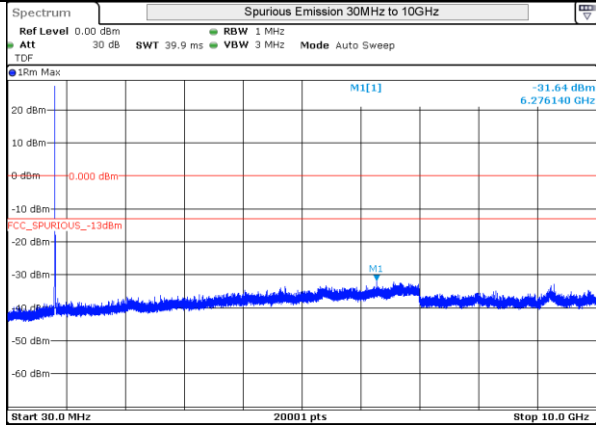
LTE 5 QPSK BW10MHz Low Ch 20450 1RB-0
