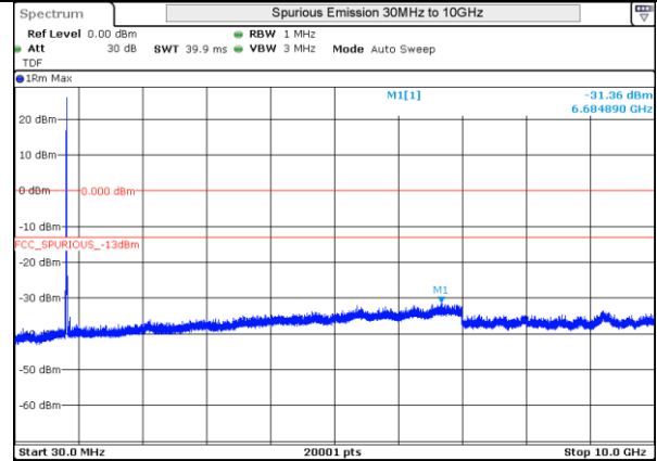
LTE 5 QPSK BW10MHz Mid Ch 20525 1RB-0
