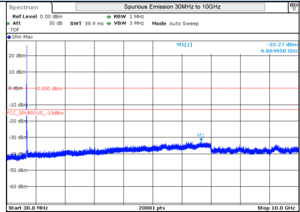
LTE 17 16QAM BW10MHz High Ch 23800 1RB-0
