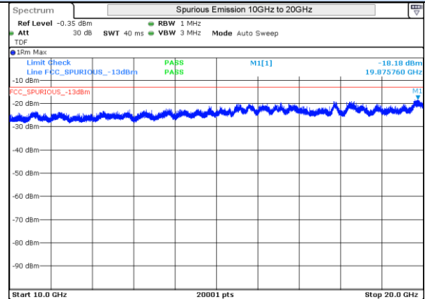
LTE 4 16QAM BW20MHz Mid Ch 20175 1RB-0
