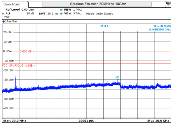
LTE 5 16QAM BW5MHz Mid Ch 20525 1RB-0
