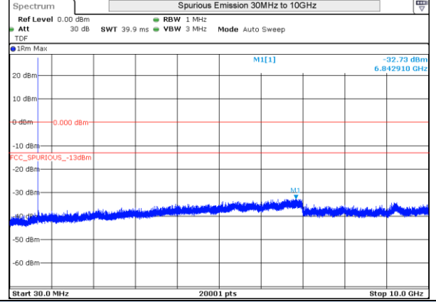
LTE 12 16QAM BW1.4MHz 699.7MHz Low ch 23017 1RB-0
