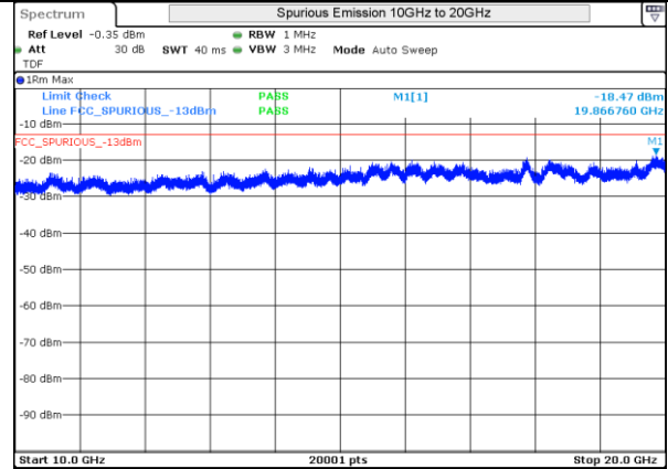
LTE 4 16QAM BW10MHz Low Ch 20000 1RB-0
