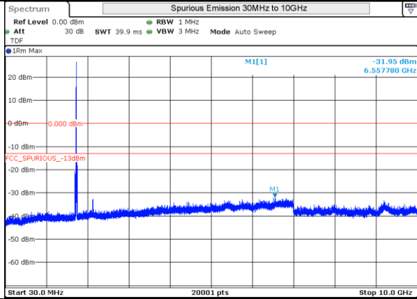
LTE 4 QPSK BW15MHz High Ch 20325 1RB-0
