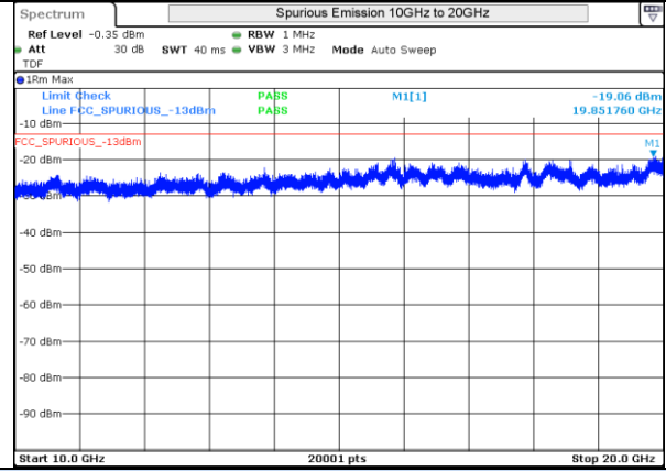
LTE 4 QPSK BW5MHz Mid Ch 20175 1RB-0
