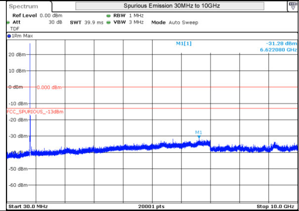
LTE 5 16QAM BW10MHz Low Ch 20450 1RB-0
