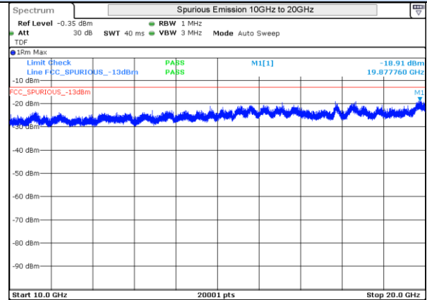
LTE 4 16QAM BW20MHz High Ch 20300 1RB-0
