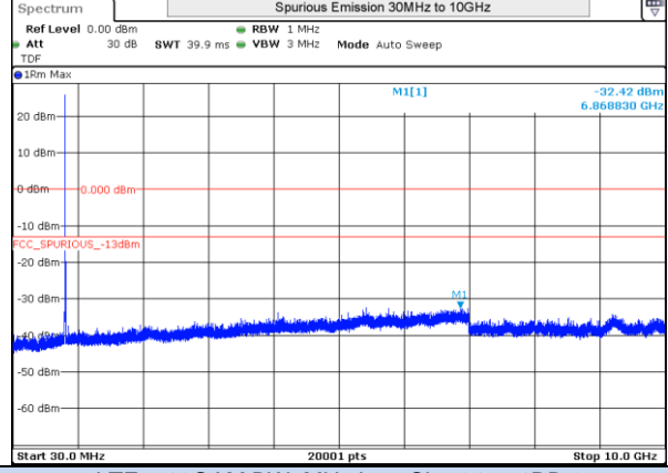
LTE 5 16QAM BW5MHz Low Ch 20425 1RB-0
