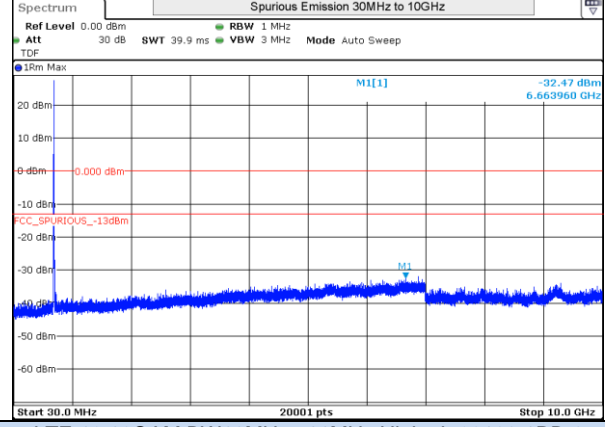
LTE 12 16QAM BW10MHz 704MHz Low ch 23060 1RB-0
