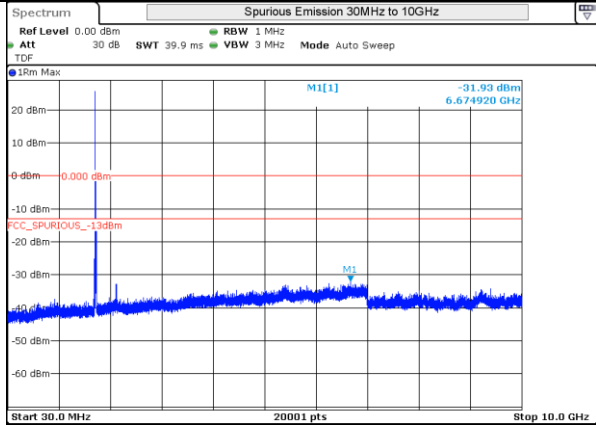
LTE 4 QPSK BW15MHz Mid Ch 20175 1RB-0
