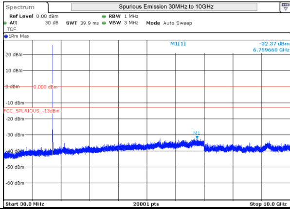
LTE 4 16QAM BW5MHz Mid Ch 20175 1RB-0
