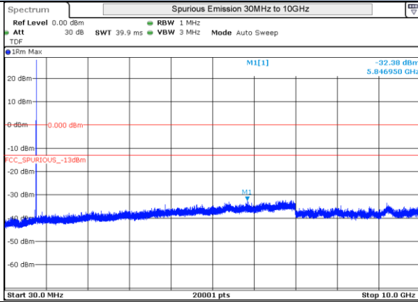
LTE 13 QPSK BW5MHz 784.5MHz High ch 23255 1RB-0
