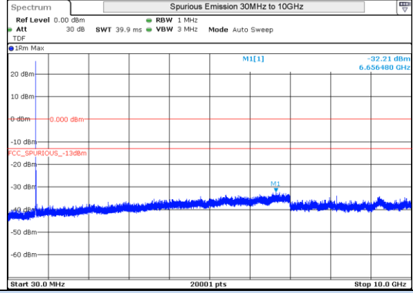
LTE 12 16QAM BW3MHz 714.5MHz High ch 23165 1RB-0
