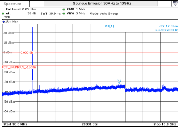
LTE 4 QPSK BW10MHz Mid Ch 20175 1RB-0
