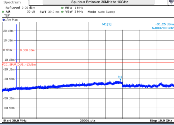
LTE 5 QPSK BW5MHz High Ch 20625 1RB-0
