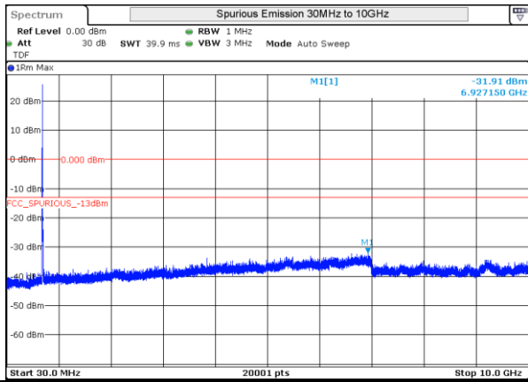
LTE 17 QPSK BW10MHz High Ch 23800 1RB-0
