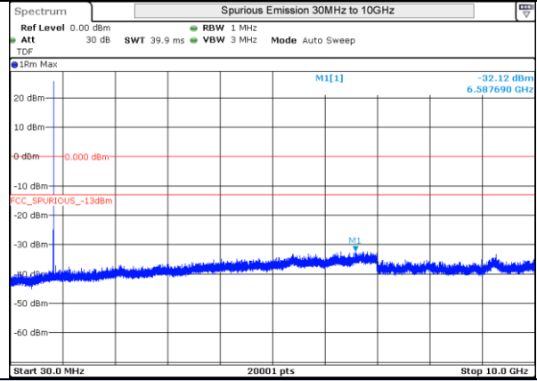
LTE 5 16QAM BW3MHz High Ch 20635 1RB-0
