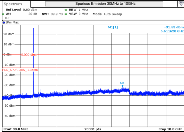
LTE 4 16QAM BW3MHz Mid Ch 20175 1RB-0
