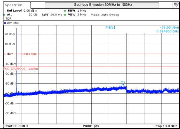
LTE 13 16QAM BW10MHz 782MHz Low ch 23230 1RB-0
