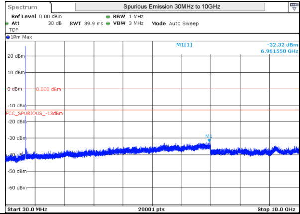
LTE 12 16QAM BW3MHz 700.5MHz Low ch 23025 1RB-0
