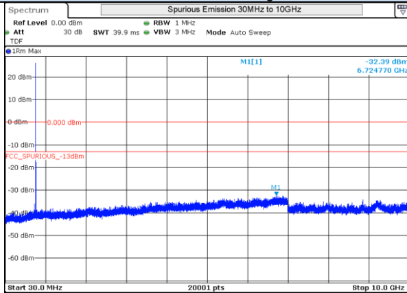
LTE 13 16QAM BW10MHz 782MHz Mid ch 23230 1RB-0
