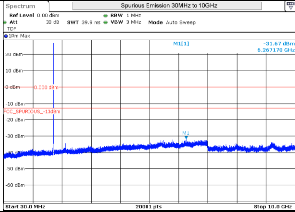
LTE 4 QPSK BW5MHz Mid Ch 20175 1RB-0
