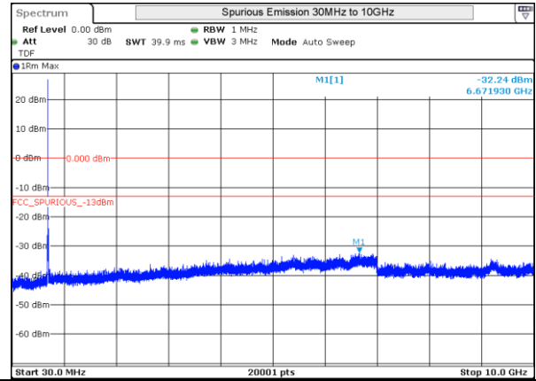
LTE 12 16QAM BW5MHz 713.5MHz High ch 23035 1RB-0
