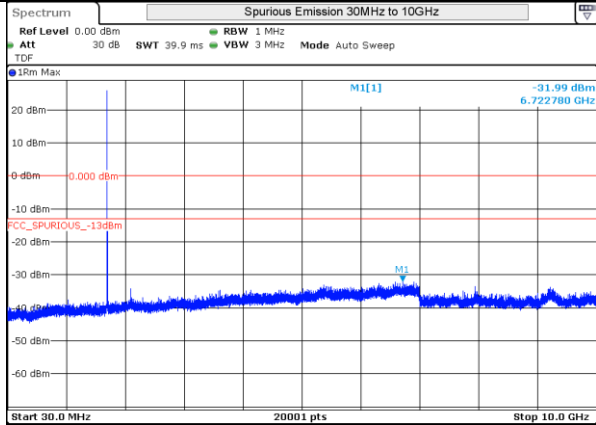
LTE 4 16QAM BW3MHz Low Ch 19965 1RB-0
