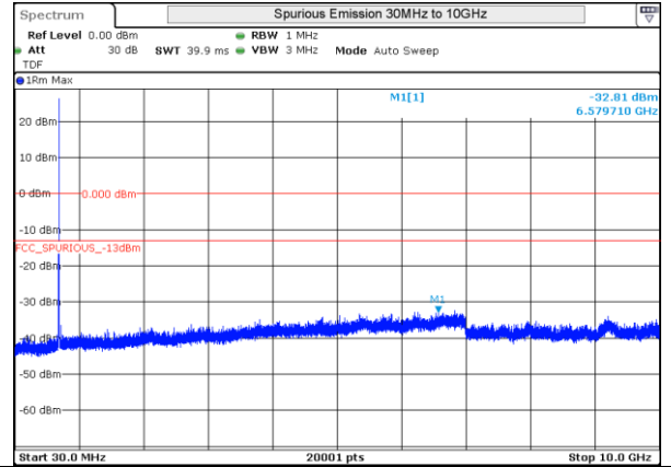
LTE 12 QPSK BW1.4MHz 707.5MHz Mid ch 23095 1RB-0
