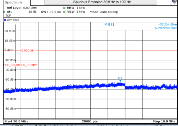
LTE 12 QPSK BW5MHz 707.5MHz Mid ch 23095 1RB-0
