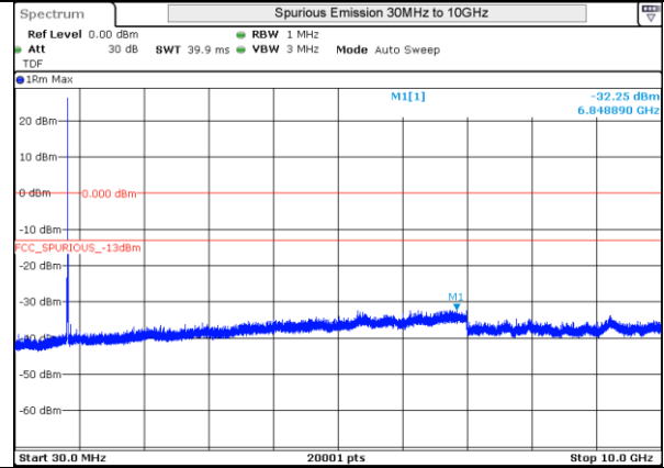
LTE 5 16QAM BW10MHz High Ch 20600 1RB-0
