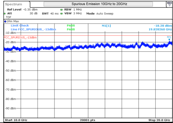
LTE 4 QPSK BW5MHz Low Ch 19975 1RB-0
