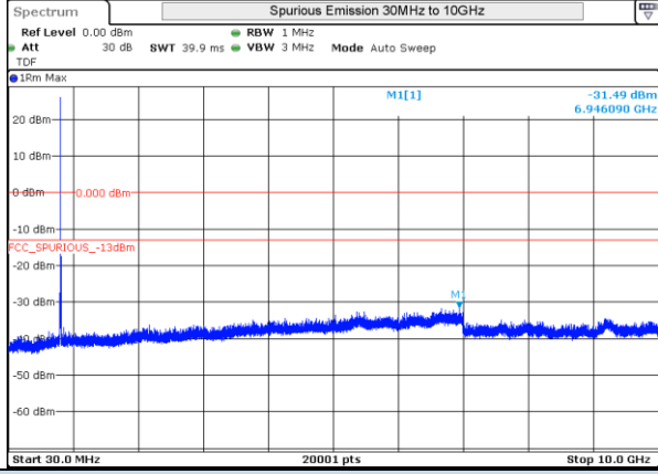
LTE 5 QPSK BW5MHz Low Ch 20425 1RB-0
