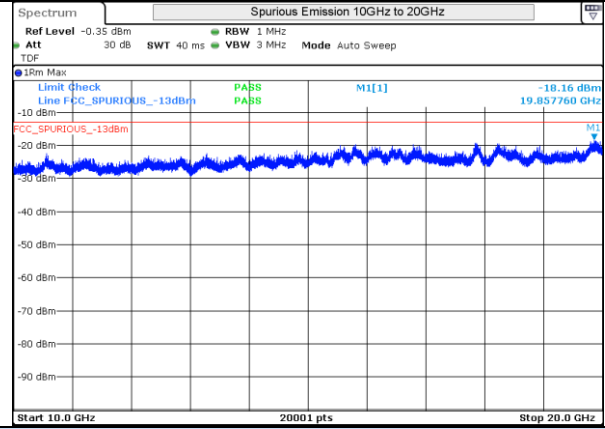
LTE 4 QPSK BW20MHz Low Ch 20050 1RB-0
