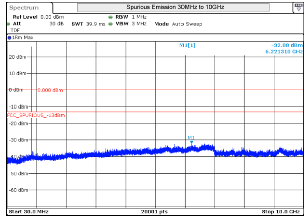
LTE 5 16QAM BW5MHz High Ch 20625 1RB-0
