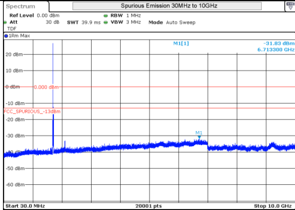
LTE 4 16QAM BW10MHz Low Ch 20000 1RB-0
