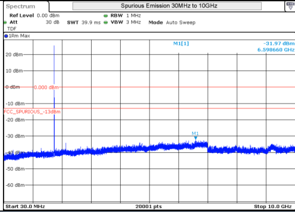
LTE 4 QPSK BW5MHz High Ch 20375 1RB-0
