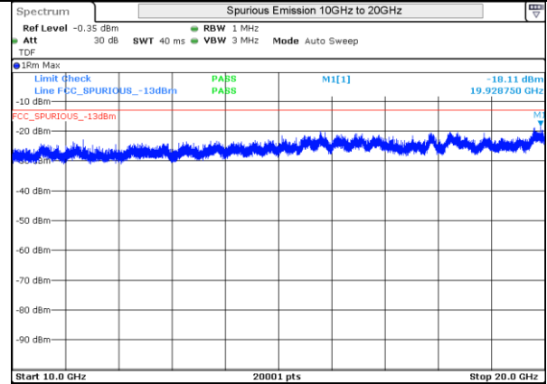
LTE 4 16QAM BW20MHz Low Ch 20050 1RB-0
