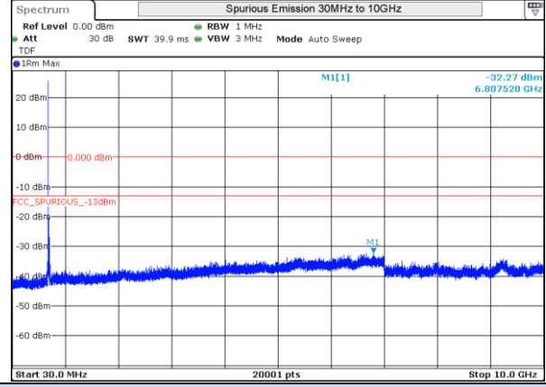
LTE 12 QPSK BW10MHz 707.5MHz Mid ch 23095 1RB-0
