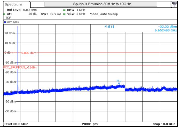
LTE 5 16QAM BW3MHz Low Ch 20415 1RB-0
