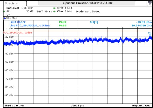
LTE 4 QPSK BW15MHz High Ch 20325 1RB-0
