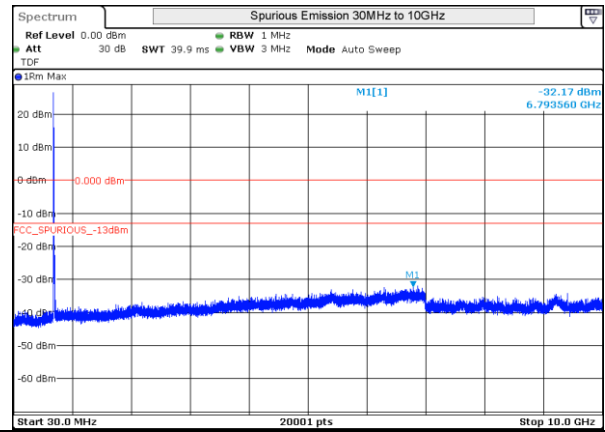
LTE 17 16QAM BW10MHz Low Ch 23780 1RB-0
