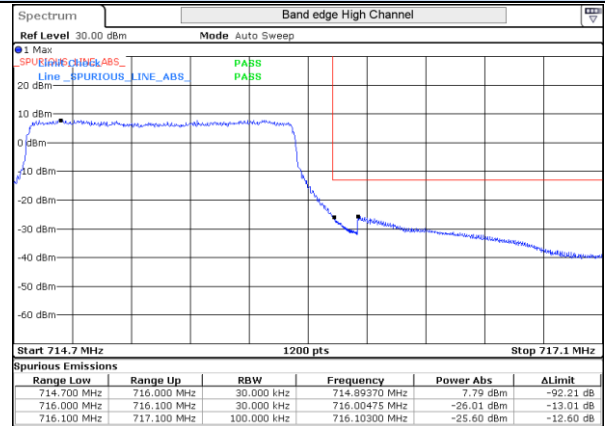
LTE 12 QPSK BW1.4MHz 715.3MHz High ch 23173 6RB-0
