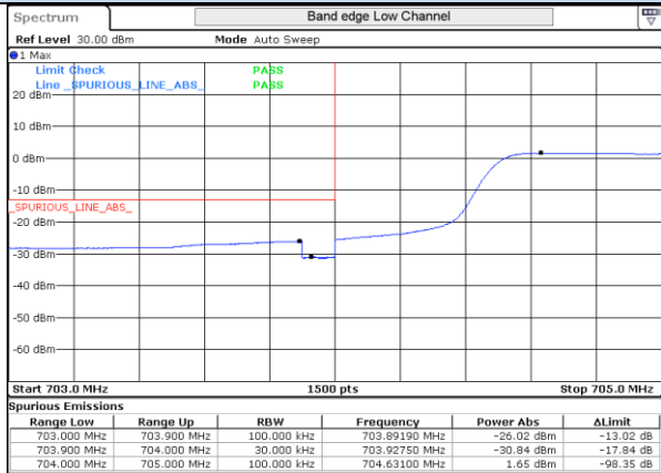
LTE 17 QPSK BW10MHz Low Ch 23780 50RB-0
