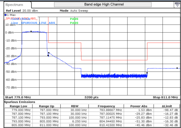
LTE 13 QPSK BW5MHz 784.5MHz High ch 23255 25RB-0
