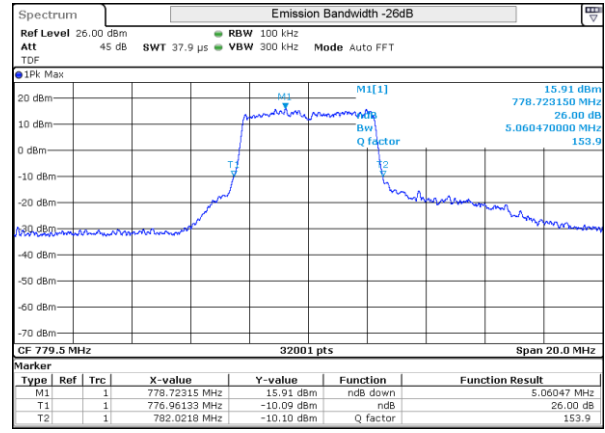
LTE 13 16QAM BW5MHz 779.5MHz Low ch 23205 25RB-0
