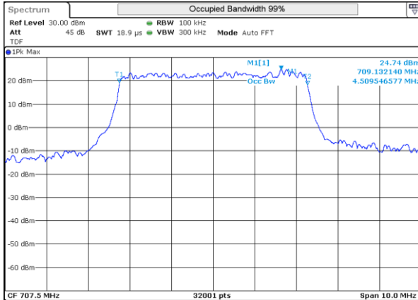
LTE 12 16QAM BW5MHz 707.5MHz Mid ch 23095 25RB-0
