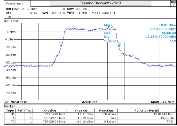
LTE 13 16QAM BW10MHz 782MHz Low ch 23230 50RB-0
