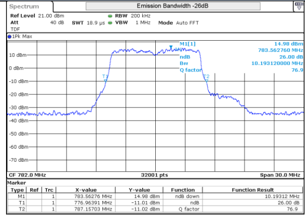
LTE 13 16QAM BW10MHz 782MHz Mid ch 23230 50RB-0
