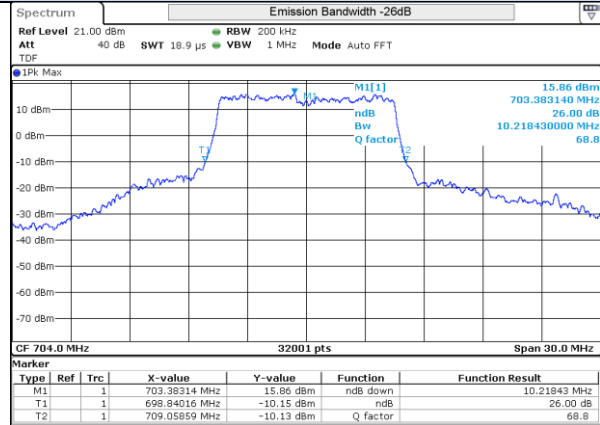
LTE 12 QPSK BW10MHz 704MHz Low ch 23060 50RB-0
