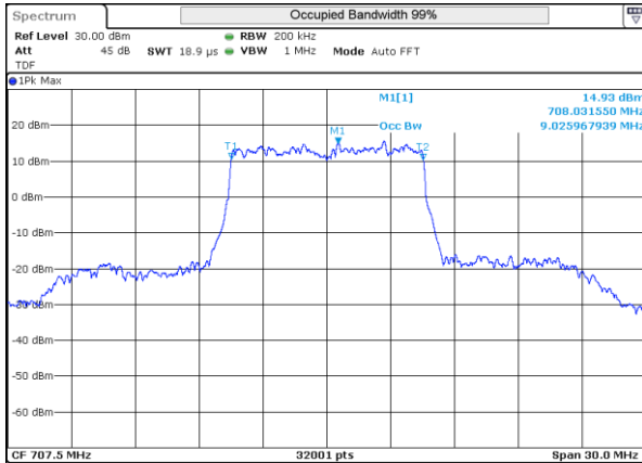
LTE 12 QPSK BW10MHz 707.5MHz Mid ch 23095 50RB-0
