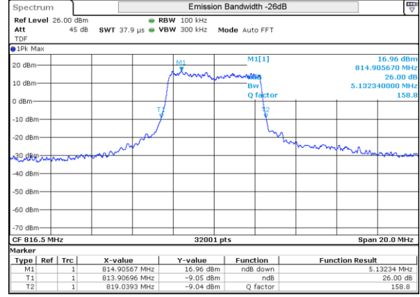
LTE 26 QPSK BW5MHz 816.5MHz Low ch 26715 25RB-0
