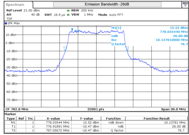
LTE 13 16QAM BW10MHz 782MHz High ch 23230 50RB-0
