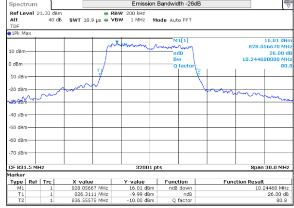
LTE 26 16QAM BW10MHz 831.5MHz Mid ch 26865 50RB-0
