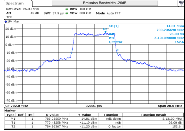
LTE 13 16QAM BW5MHz 782MHz Mid ch 23230 25RB-0
