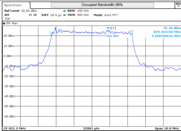
LTE 26 QPSK BW5MHz 831.5MHz Mid ch 26865 25RB-0
