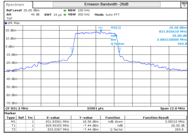
LTE 26 QPSK BW3MHz 831.5MHz Mid ch 26865 15RB-0
