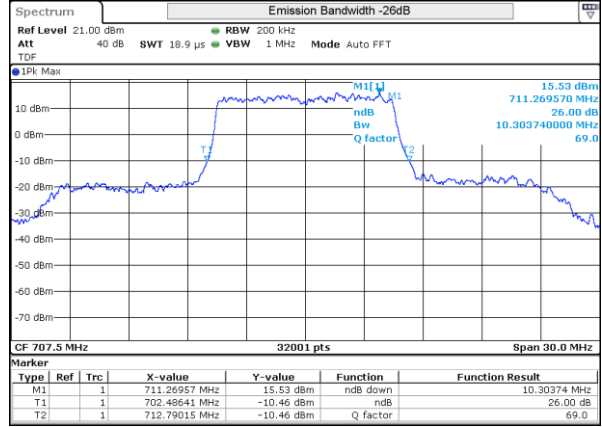
LTE 12 QPSK BW10MHz 707.5MHz Mid ch 23095 50RB-0
