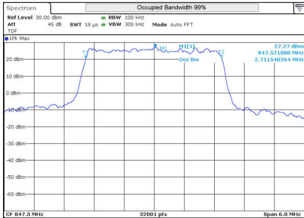
LTE 26 QPSK BW3MHz 847.5MHz High ch 27025 15RB-0
