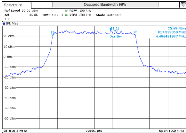
LTE 26 QPSK BW5MHz 816.5MHz Low ch 26715 25RB-0
