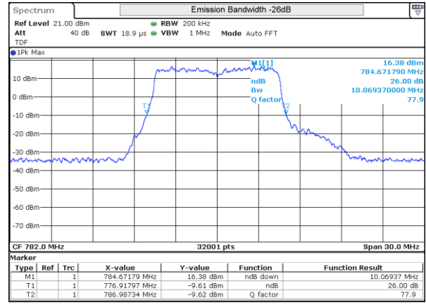
LTE 13 QPSK BW10MHz 782MHz Mid ch 23230 50RB-0
