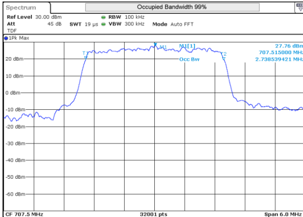
LTE 12 QPSK BW3MHz 707.5MHz Mid ch 23095 15RB-0
