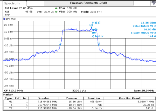
LTE 12 16QAM BW5MHz 713.5MHz High ch 23155 25RB-0
