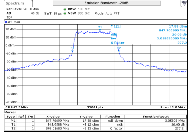
LTE 26 QPSK BW3MHz 847.5MHz High ch 27025 15RB-0
