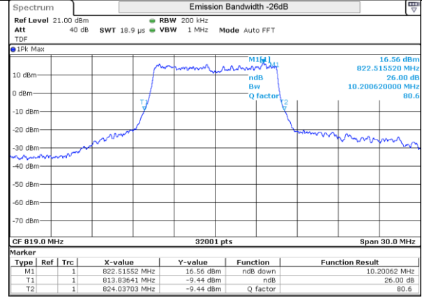
LTE 26 QPSK BW10MHz 819MHz Low ch 26740 50RB-0
