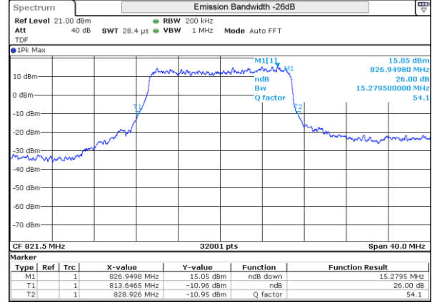
LTE 26 QPSK BW15MHz 821.5MHz Low ch 26765 75RB-0
