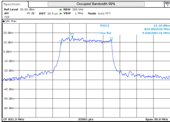
LTE 26 16QAM BW10MHz 831.5MHz Mid ch 26865 50RB-0
