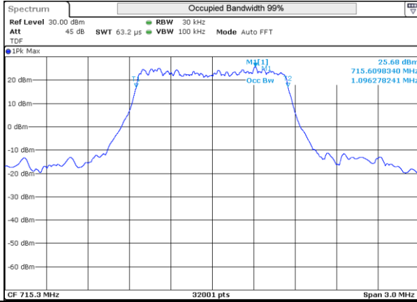
LTE 12 16QAM BW1.4MHz 715.3MHz Mid ch 23173 6RB-0
