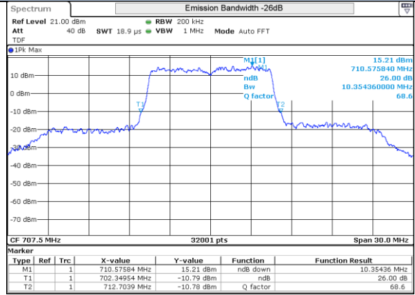
LTE 12 16QAM BW10MHz 707.5MHz Mid ch 23095 50RB-0
