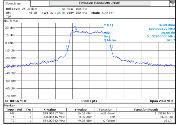
LTE 26 QPSK BW5MHz 831.5MHz Mid ch 26865 25RB-0
