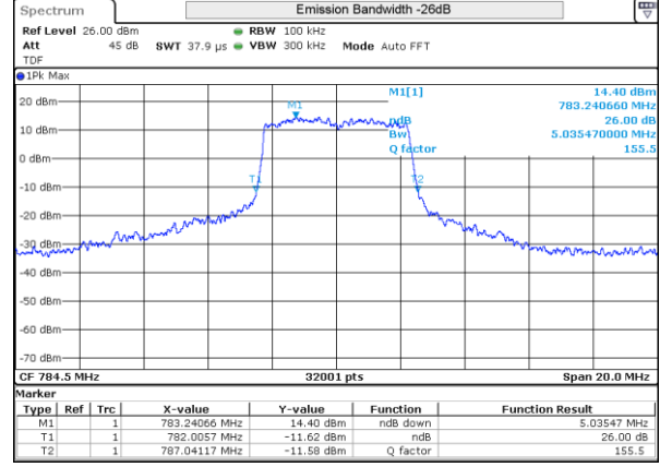
LTE 13 16QAM BW5MHz 784.5MHz High ch 23255 25RB-0
