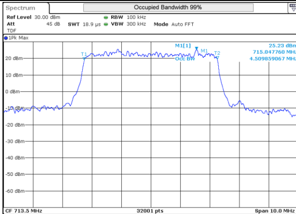
LTE 12 16QAM BW5MHz 713.5MHz High ch 23155 25RB-0
