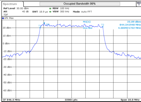
LTE 26 QPSK BW5MHz 846.5MHz High ch 27015 25RB-0
