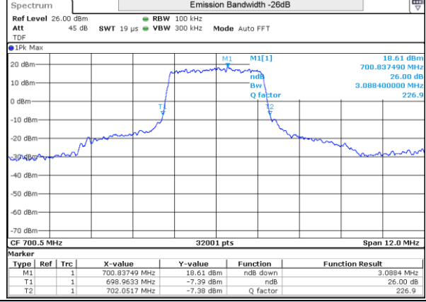
LTE 12 QPSK BW3MHz 700.5MHz Low ch 23025 15RB-0
