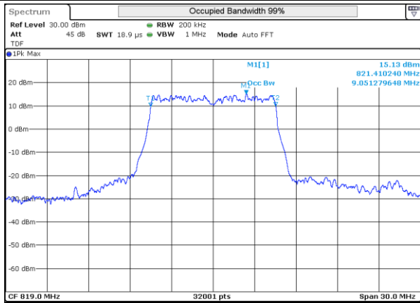
LTE 26 QPSK BW10MHz 819MHz Low ch 26740 50RB-0
