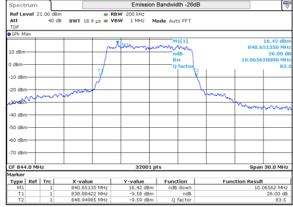
LTE 26 QPSK BW10MHz 844MHz High ch 26990 50RB-0
