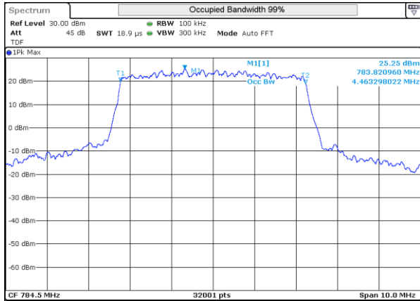
LTE 13 16QAM BW5MHz 784.5MHz High ch 23255 25RB-0
