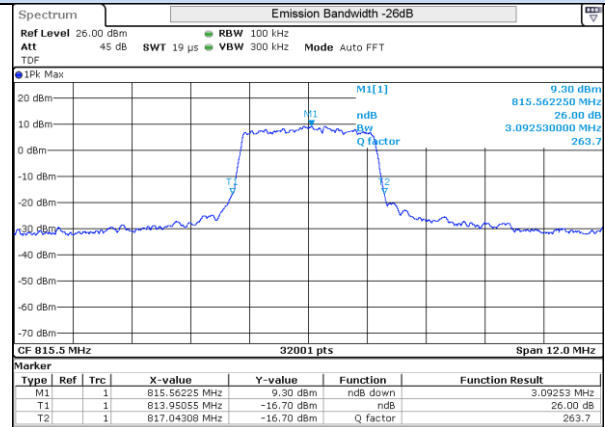
LTE 26 QPSK BW3MHz 815.5MHz Low ch 26705 15RB-0
