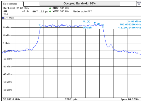
LTE 13 16QAM BW5MHz 782MHz Mid ch 23230 25RB-0
