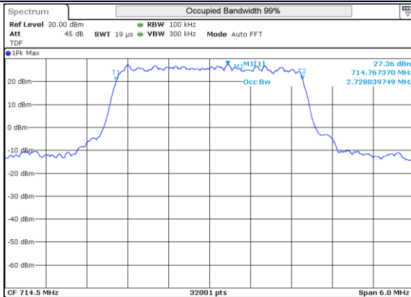
LTE 12 QPSK BW3MHz 714.5MHz Mid ch 23165 15RB-0
