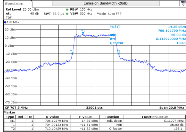
LTE 12 16QAM BW5MHz 707.5MHz Mid ch 23095 25RB-0
