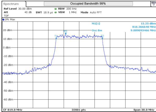
LTE 26 16QAM BW10MHz 819MHz Low ch 26740 50RB-0
