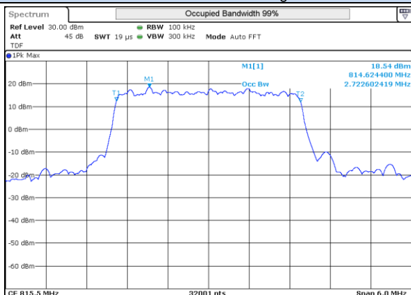
LTE 26 QPSK BW3MHz 815.5MHz Low ch 26705 15RB-0
