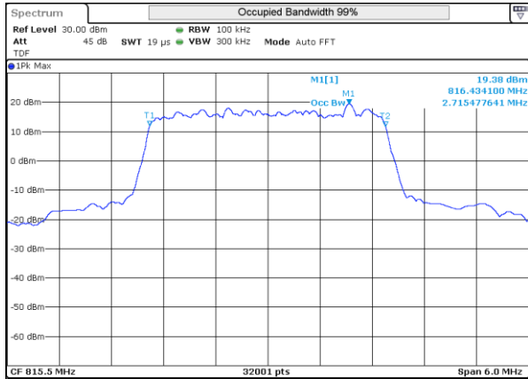
LTE 26 QPSK BW3MHz 815.5MHz High ch 27025 15RB-0
