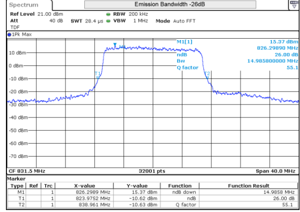
LTE 26 QPSK BW15MHz 831.5MHz Mid ch 26865 75RB-0
