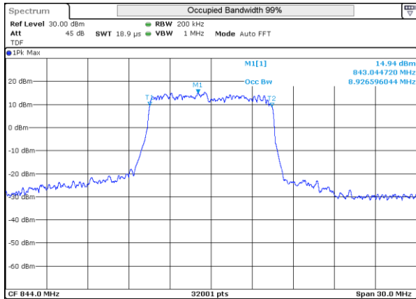
LTE 26 QPSK BW10MHz 844MHz High ch 26990 50RB-0
