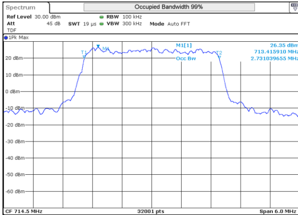
LTE 12 16QAM BW3MHz 714.5MHz High ch 23165 15RB-0
