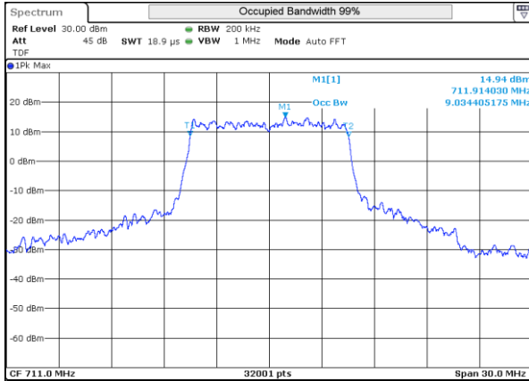
LTE 12 QPSK BW10MHz 711MHz High ch 23130 50RB-0
