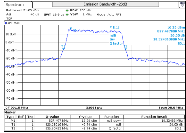
LTE 26 QPSK BW10MHz 831.5MHz Mid ch 26865 50RB-0
