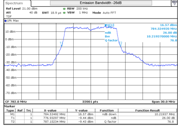
LTE 13 QPSK BW10MHz 782MHz High ch 23230 50RB-0
