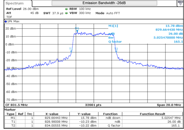
LTE 26 16QAM BW5MHz 831.5MHz Mid ch 26865 25RB-0
