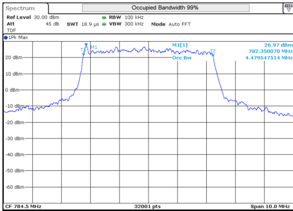
LTE 13 QPSK BW5MHz 784.5MHz High ch 23255 25RB-0
