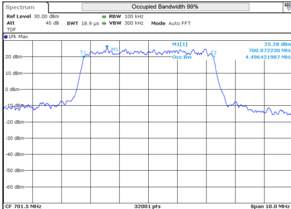
LTE 12 16QAM BW5MHz 701.5MHz Low ch 23035 25RB-0
