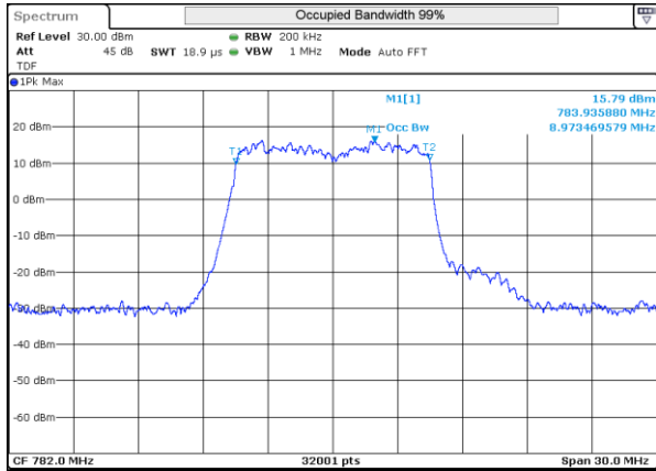
LTE 13 QPSK BW10MHz 782MHz Low ch 23230 50RB-0
