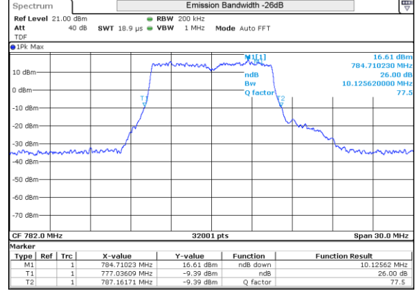
LTE 13 QPSK BW10MHz 782MHz Low ch 23230 50RB-0
