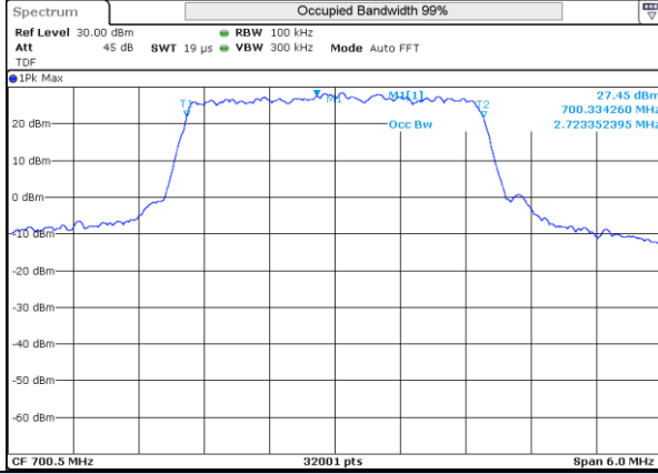
LTE 12 QPSK BW3MHz 700.5MHz Low ch 23025 15RB-0
