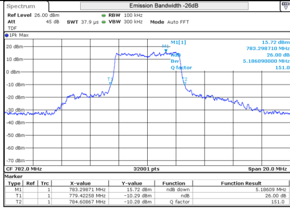
LTE 13 QPSK BW5MHz 782MHz Mid ch 23230 25RB-0
