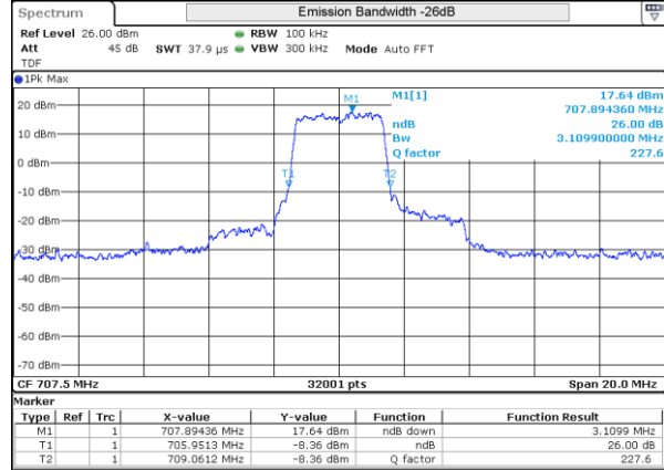
LTE 12 QPSK BW3MHz 707.5MHz Mid ch 23095 15RB-0
