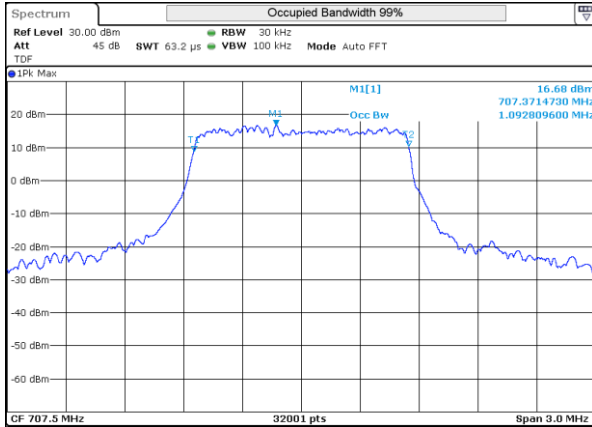
LTE 12 16QAM BW1.4MHz 707.5MHz Low ch 23095 6RB-0
