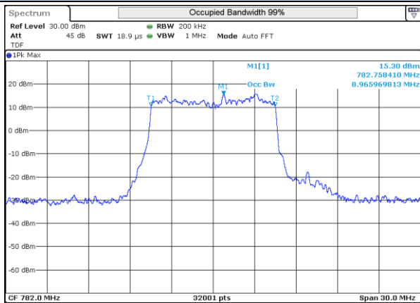
LTE 13 16QAM BW10MHz 782MHz Mid ch 23230 50RB-0
