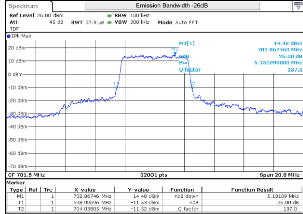
LTE 12 16QAM BW5MHz 701.5MHz Low ch 23035 25RB-0
