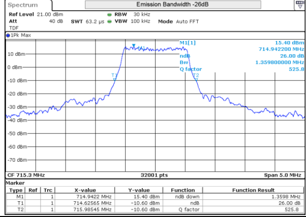
LTE 12 16QAM BW1.4MHz 715.3MHz Mid ch 23173 6RB-0
