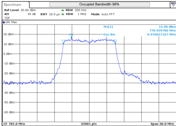
LTE 13 QPSK BW10MHz 782MHz High ch 23230 50RB-0
