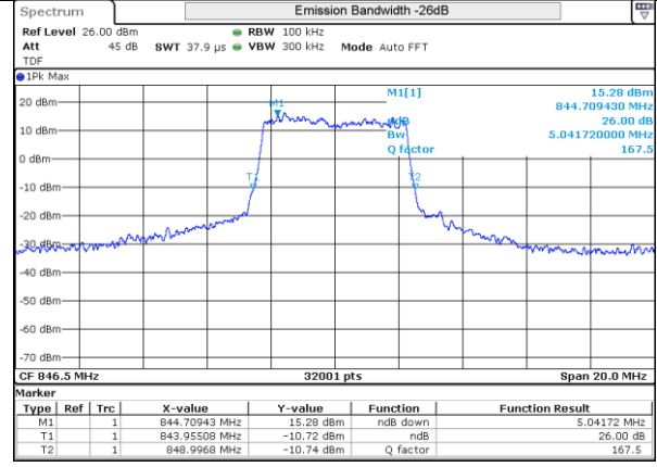
LTE 26 QPSK BW5MHz 846.5MHz High ch 27015 25RB-0
