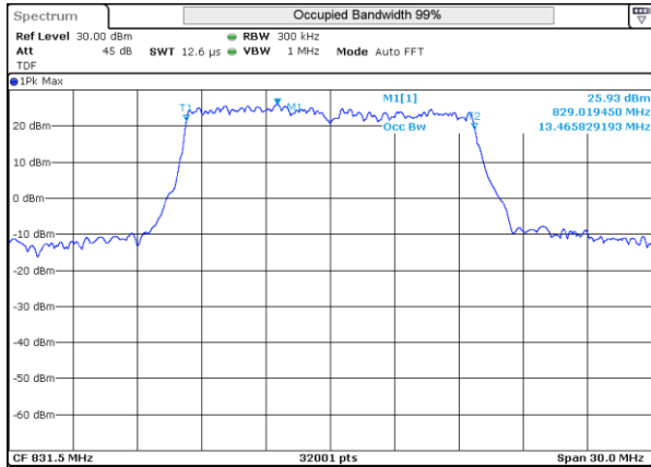
LTE 26 QPSK BW15MHz 831.5MHz Mid ch 26865 75RB-0
