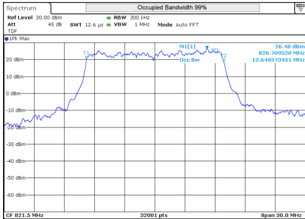
LTE 26 QPSK BW15MHz 821.5MHz Low ch 26765 75RB-0
