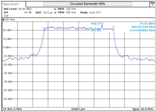
LTE 26 16QAM BW5MHz 831.5MHz Mid ch 26865 25RB-0
