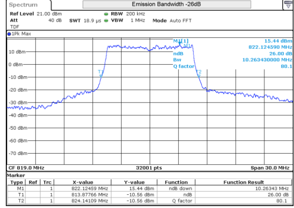
LTE 26 16QAM BW10MHz 819MHz Low ch 26740 50RB-0
