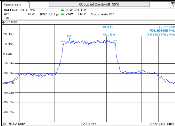
LTE 12 16QAM BW10MHz 707.5MHz Mid ch 23095 50RB-0
