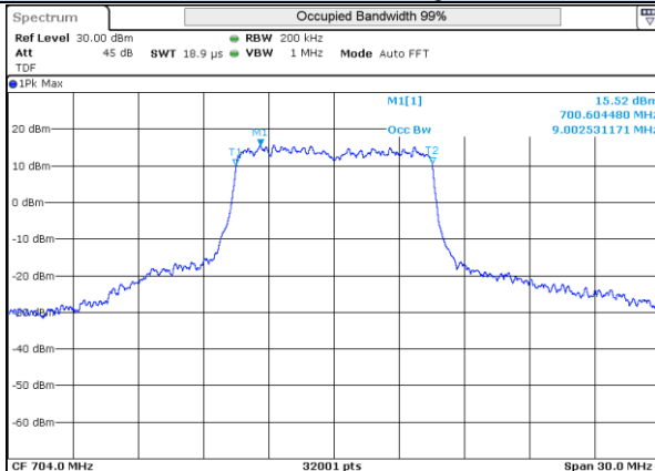
LTE 12 QPSK BW10MHz 704MHz Low ch 23060 50RB-0
