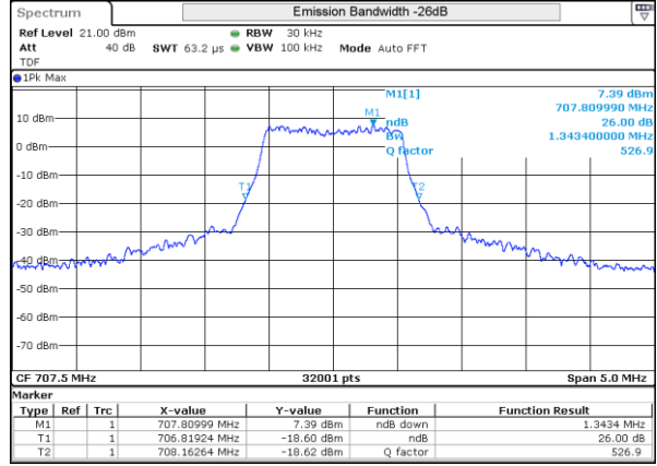
LTE 12 16QAM BW1.4MHz 707.5MHz Low ch 23095 6RB-0
