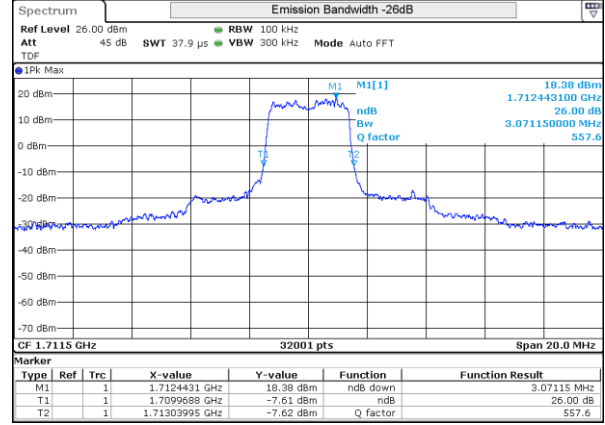
LTE 4 QPSK BW3MHz Low ch 19965 15RB-0
