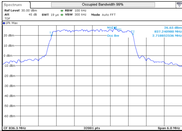
LTE 5 16QAM BW3MHz Mid ch 20525 15RB-0
