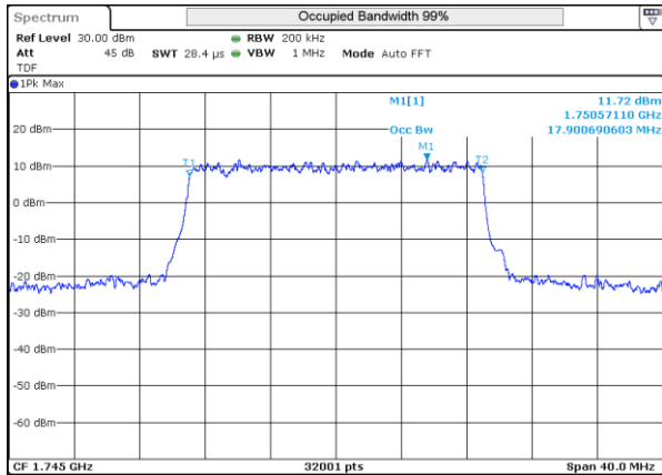
LTE 4 16QAM BW20MHz High ch 20300 100RB-0
