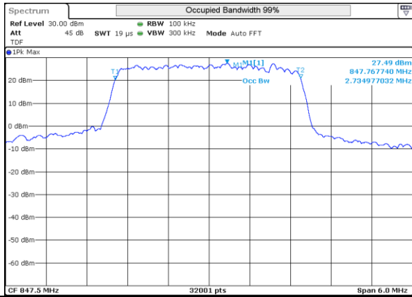
LTE 5 QPSK BW3MHz High ch 20635 15RB-0
