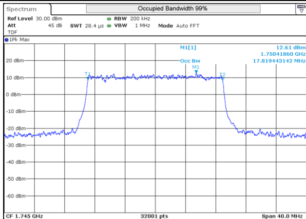
LTE 4 QPSK BW20MHz High ch 20300 100RB-0
