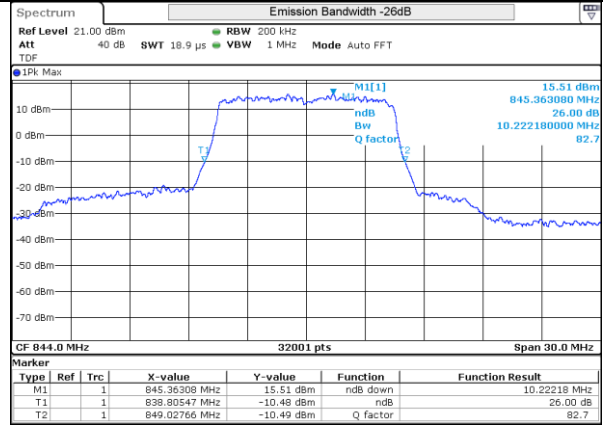
LTE 5 QPSK BW10MHz High ch 20600 50RB-0
