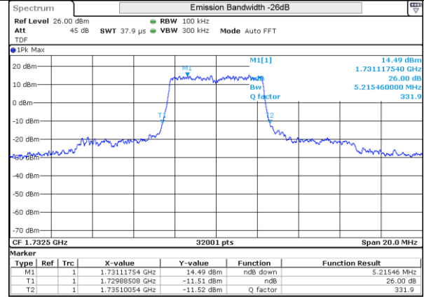
LTE 4 QPSK BW5MHz Mid ch 20175 25RB-0
