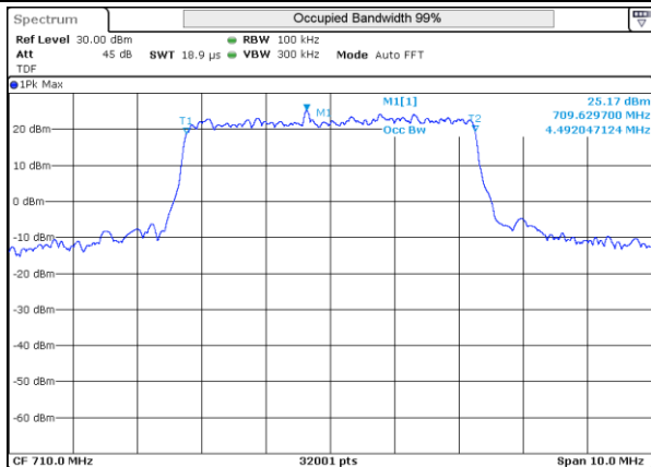
LTE 17 16QAM BW5MHz Mid ch 23790 25RB-0
