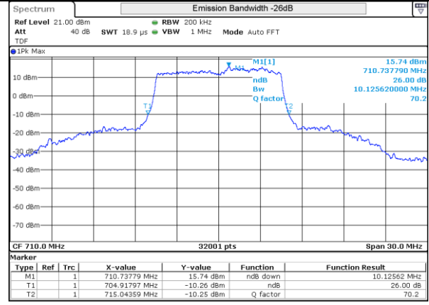
LTE 17 16QAM BW10MHz Mid ch 23790 50RB-0
