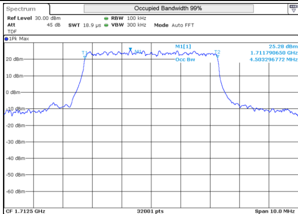
LTE 4 QPSK BW5MHz Low ch 19975 25RB-0
