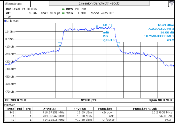
LTE 17 QPSK BW10MHz Low ch 23780 50RB-0
