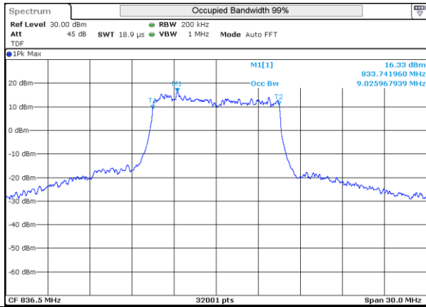
LTE 5 16QAM BW10MHz Mid ch 20525 50RB-0
