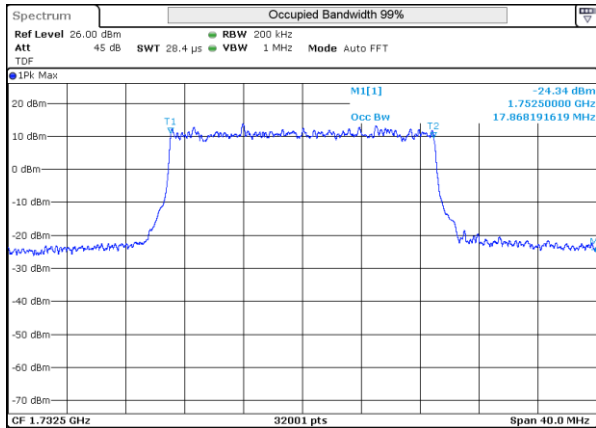
LTE 4 QPSK BW20MHz Mid ch 20175 100RB-0
