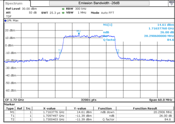
LTE 4 16QAM BW20MHz Low ch 20050 100RB-0
