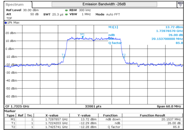
LTE 4 QPSK BW20MHz Mid ch 20175 100RB-0
