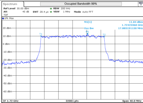
LTE 4 16QAM BW20MHz Low ch 20050 100RB-0
