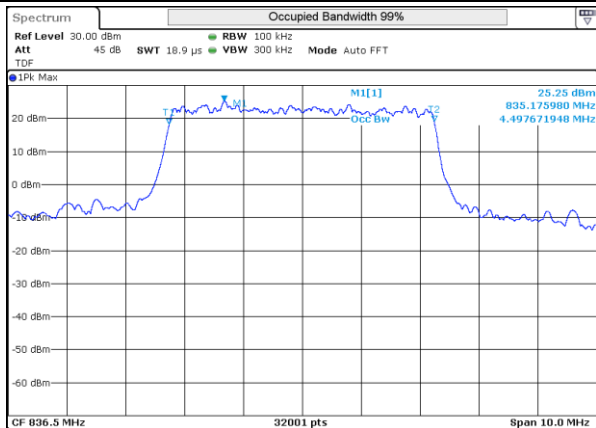
LTE 5 16QAM BW5MHz Mid ch 20525 25RB-0
