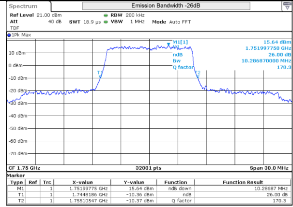
LTE 4 QPSK BW10MHz High ch 20350 50RB-0
