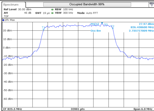
LTE 5 QPSK BW3MHz Low ch 20415 15RB-0
