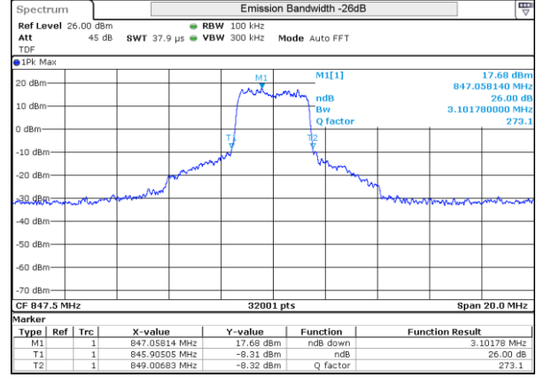
LTE 5 QPSK BW3MHz High ch 20635 15RB-0
