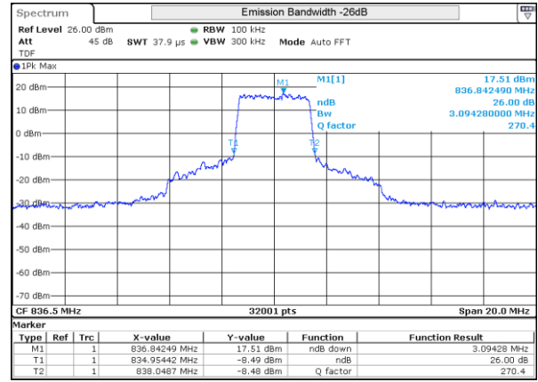
LTE 5 QPSK BW3MHz Mid ch 20525 15RB-0
