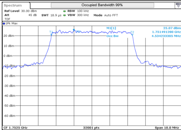
LTE 4 QPSK BW5MHz High ch 20375 25RB-0
