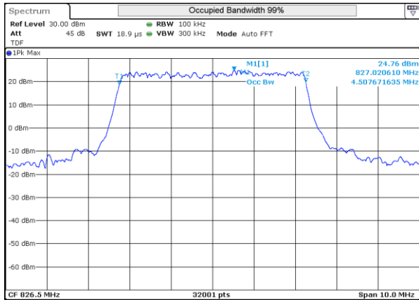
LTE 5 QPSK BW5MHz Low ch 20425 25RB-0
