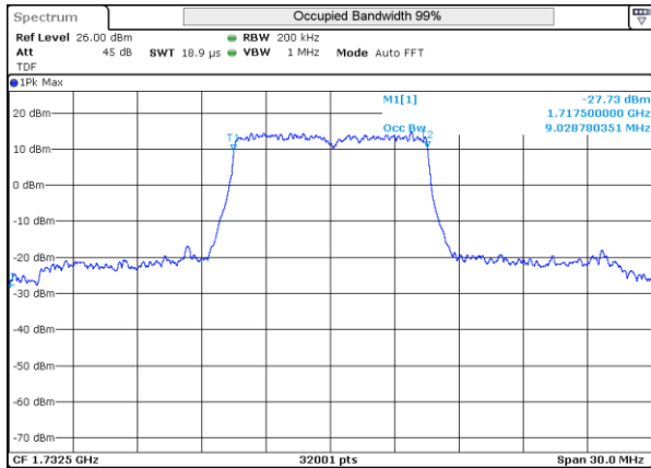
LTE 4 QPSK BW10MHz Mid ch 20175 50RB-0
