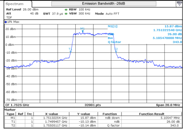
LTE 4 QPSK BW5MHz High ch 20375 25RB-0
