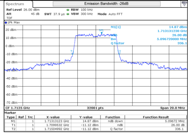
LTE 4 QPSK BW5MHz Low ch 19975 25RB-0
