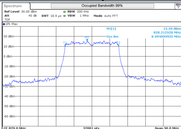
LTE 5 QPSK BW10MHz Low ch 20450 50RB-0
