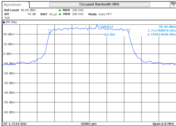
LTE 4 QPSK BW3MHz Low ch 19965 15RB-0
