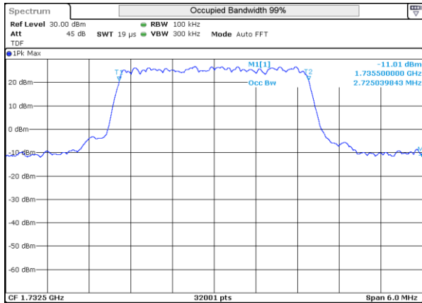
LTE 4 QPSK BW3MHz Mid ch 20175 15RB-0
