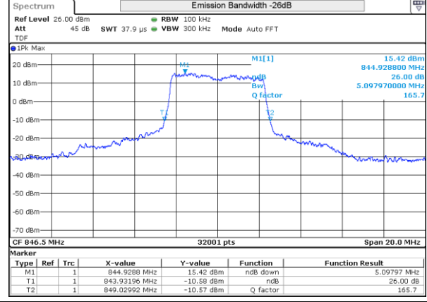
LTE 5 QPSK BW5MHz High ch 20625 25RB-0
