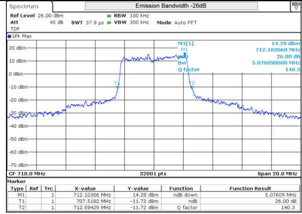
LTE 17 16QAM BW5MHz Mid ch 23790 25RB-0
