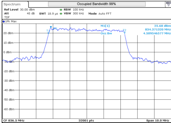
LTE 5 QPSK BW5MHz Mid ch 20525 25RB-0
