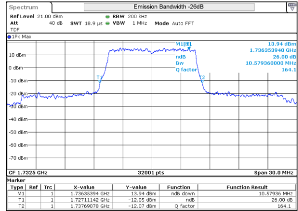
LTE 4 QPSK BW10MHz Mid ch 20175 50RB-0
