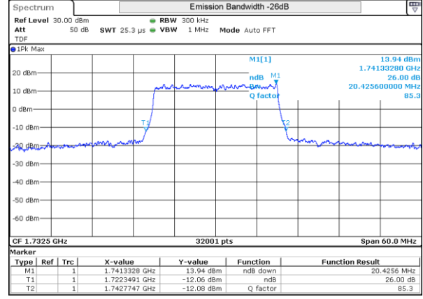
LTE 4 16QAM BW20MHz Mid ch 20175 100RB-0
