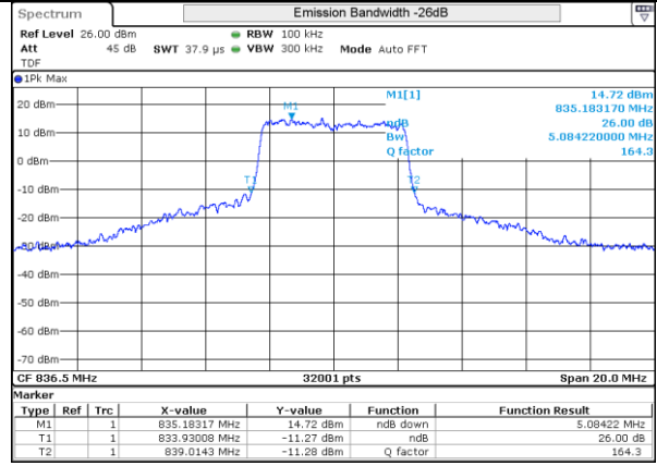
LTE 5 16QAM BW5MHz Mid ch 20525 25RB-0
