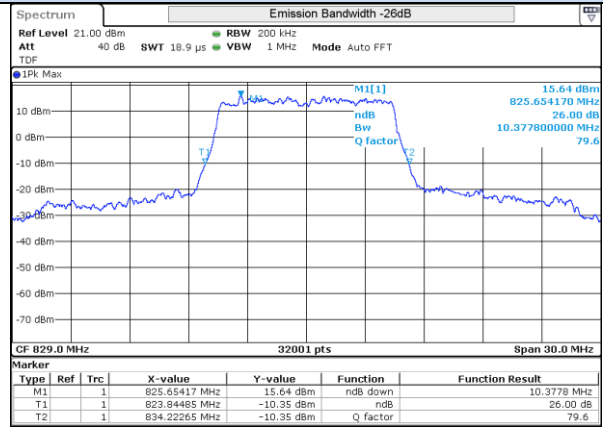
LTE 5 QPSK BW10MHz Low ch 20450 50RB-0
