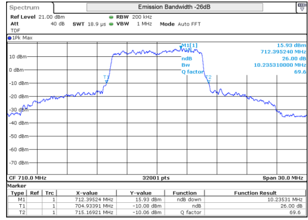
LTE 17 QPSK BW10MHz Mid ch 23790 50RB-0
