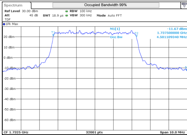
LTE 4 QPSK BW5MHz Mid ch 20175 25RB-0
