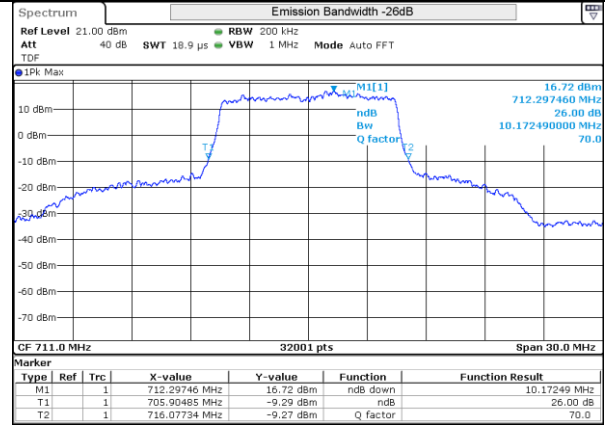
LTE 17 QPSK BW10MHz High ch 23800 50RB-0
