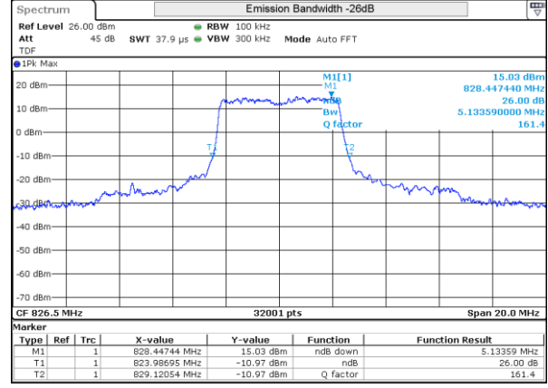
LTE 5 QPSK BW5MHz Low ch 20425 25RB-0
