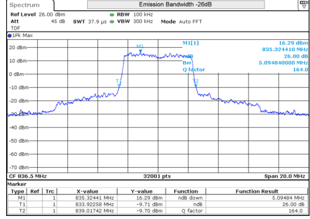
LTE 5 QPSK BW5MHz Mid ch 20525 25RB-0
