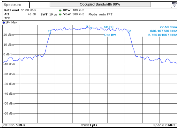
LTE 5 QPSK BW3MHz Mid ch 20525 15RB-0
