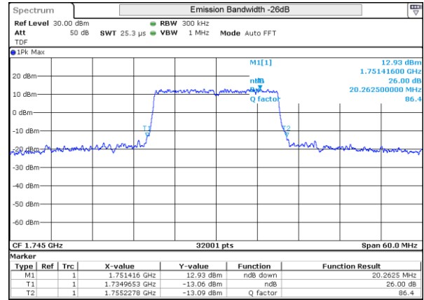
LTE 4 16QAM BW20MHz High ch 20300 100RB-0
