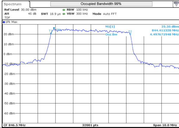
LTE 5 QPSK BW5MHz High ch 20625 25RB-0
