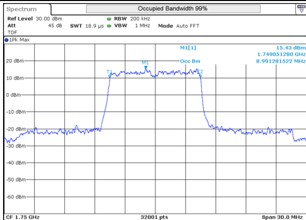
LTE 4 QPSK BW10MHz High ch 20350 50RB-0
