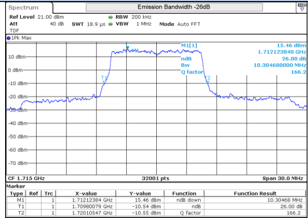
LTE 4 QPSK BW10MHz Low ch 20000 50RB-0
