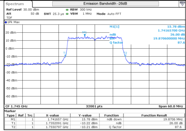
LTE 4 QPSK BW20MHz High ch 20300 100RB-0
