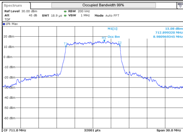
LTE 17 QPSK BW10MHz High ch 23800 50RB-0
