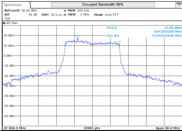
LTE 5 QPSK BW10MHz Mid ch 20525 50RB-0
