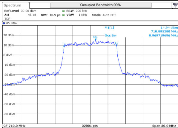
LTE 17 16QAM BW10MHz Mid ch 23790 50RB-0
