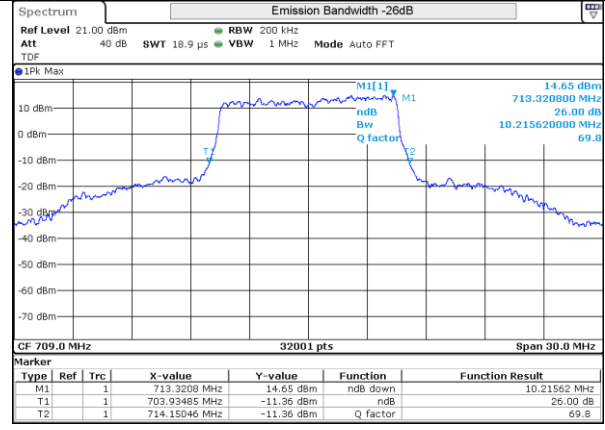
LTE 17 16QAM BW10MHz Low ch 23780 50RB-0
