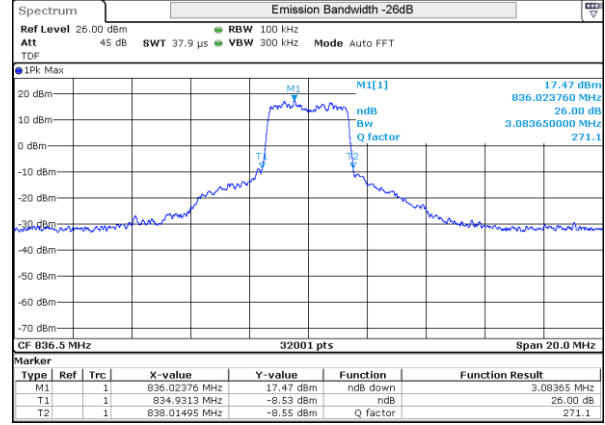
LTE 5 16QAM BW3MHz Mid ch 20525 15RB-0
