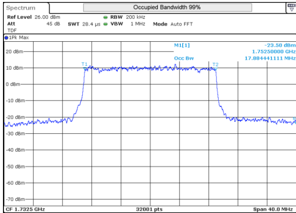
LTE 4 16QAM BW20MHz Mid ch 20175 100RB-0
