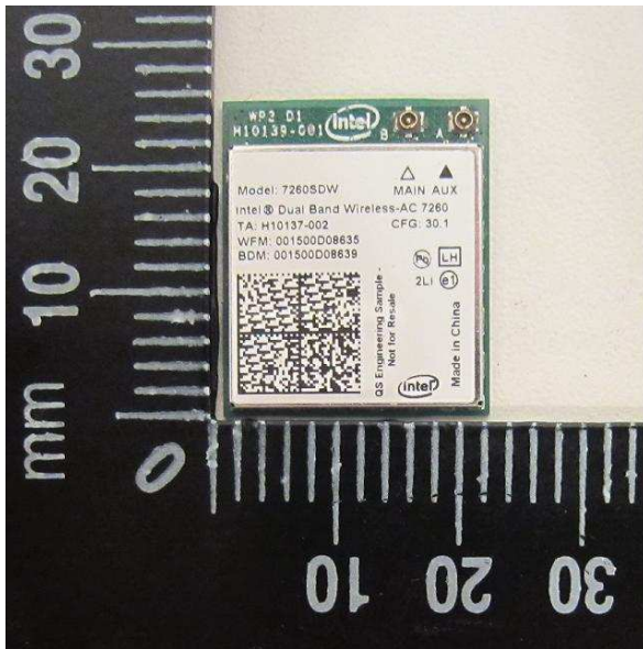
Fig. 1. Module frontal view
